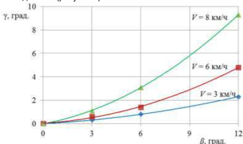
Рисунок 4 – Зависимость угла наклона кузова ПТРС-2 от угла уклона поля и скорости движения ПТРС-2
