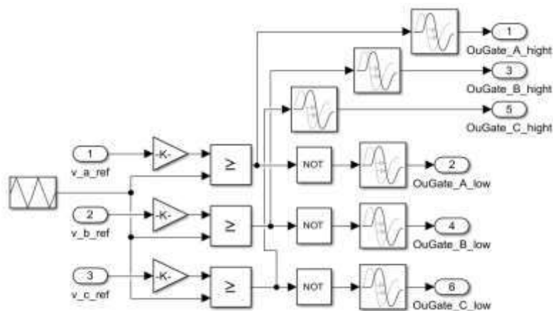
Рисунок 6 – Подсистема SPWM модулятора Figure 6 – SPWM modulator subsystem
