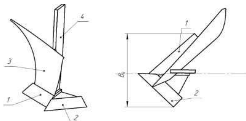
Рисунок 3 – Конструктивно-технологическая схема нового корпуса плуга общего назначения: 1 – лемех правый; 2 – лемех левый; 3 – отвал; 4 – стойка; B_k – ширина захвата корпуса плуга Figure 3 – Design and technological scheme of a new general-purpose plough body: 1 – right share; 2 – left share; 3 – blade; 4 – post; B_k – plough body width
