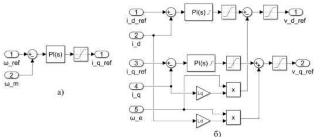
Рисунок 4 – Структура контуров регулирования скорости и тока: а) подсистема регулятора скорости; б) подсистема токовых регуляторов Figure 4 – Structure of speed and current control loops: а) speed regulator subsystem; b) subsystem of current regulators
