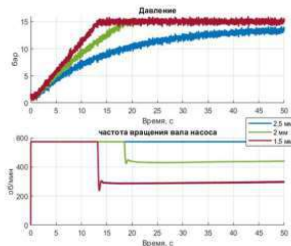
Рисунок 9 – Зависимости давления и частоты вращения вала насоса от времени при разном проходном сечении сопла форсунки при уставке давления 15 бар Figure 9 – The dependence of the pressure and speed of rotation of the pump shaft on time at different flow sections of the injector nozzle at a pressure setpoint of 15 bar
