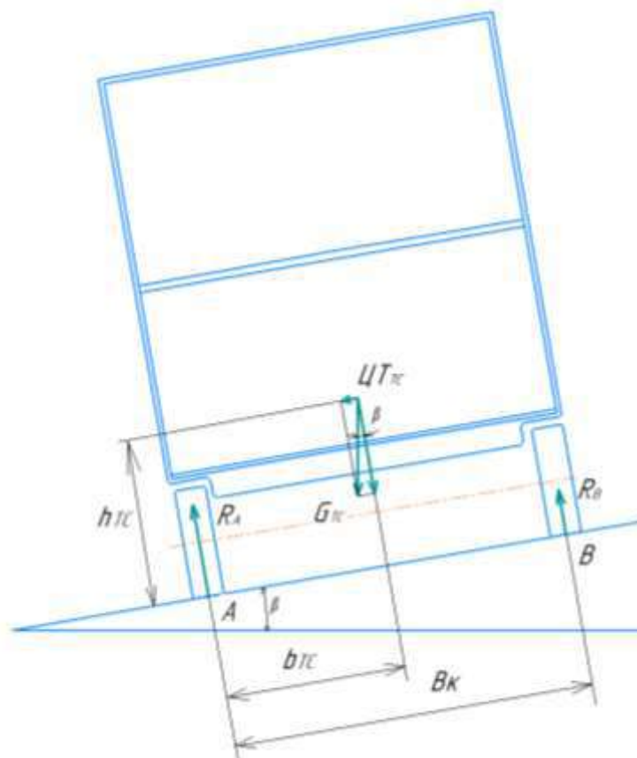
Рисунок 2 – Схема сил, действующих на подборщик-транспортировщик рулонов сена при стационарном его положении на площадке с поперечным уклоном Figure 2 – Diagram of forces acting on the hay roll picker-transporter at its stationary position on the site with a transverse slope
