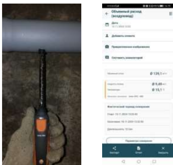
Рисунок 6 – Измерение расхода воздуха Figure 6 – Air flow measurement
