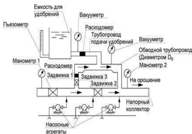
Рисунок 1 – Схема ввода удобрений в напорный трубопровод насосной станции в ЗАО «Нива»
