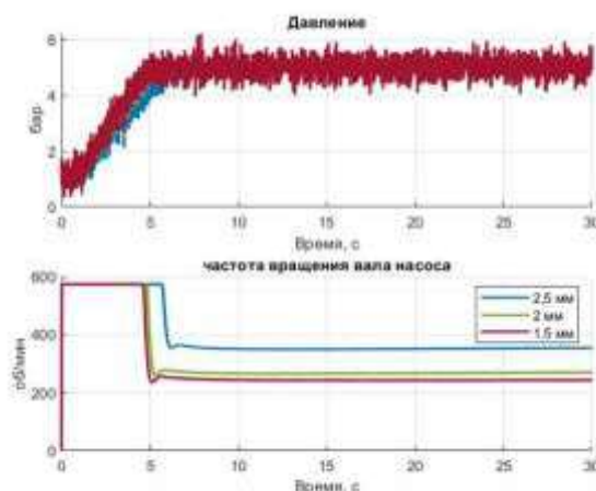
Рисунок 7 – Зависимости давления и частоты вращения вала насоса от времени при разном проходном сечении сопла форсунки при уставке давления 5 бар
