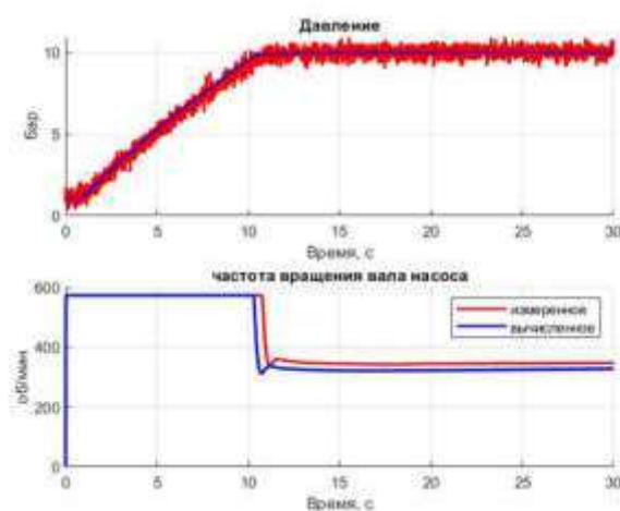
Рисунок 6 – Зависимости давления пара и частоты вращения вала насоса измеренных и вычисленных от времени
