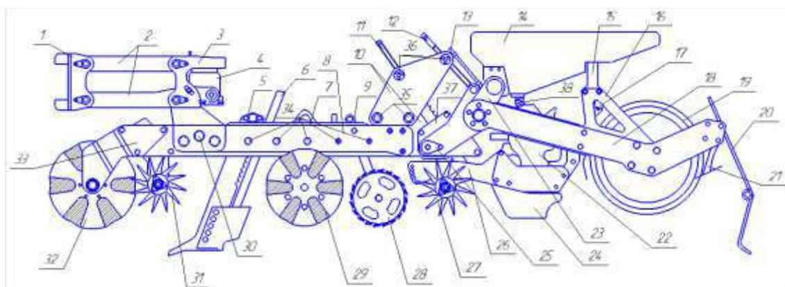
Рисунок 1 – Комбинированная секция для полосовой обработки почвы и посева сельскохозяйственных культур
