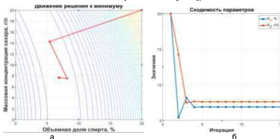
Рисунок 4 – Контурная карта функции невязки (а) и график сходимости параметров (б) при X_1 = 7\% и X_2 = 7 г/л Figure 4 – Contour map of the residual function (a) and parameter convergence graph (b) at X_1 = 7\% and X_2 = 7 g/l
