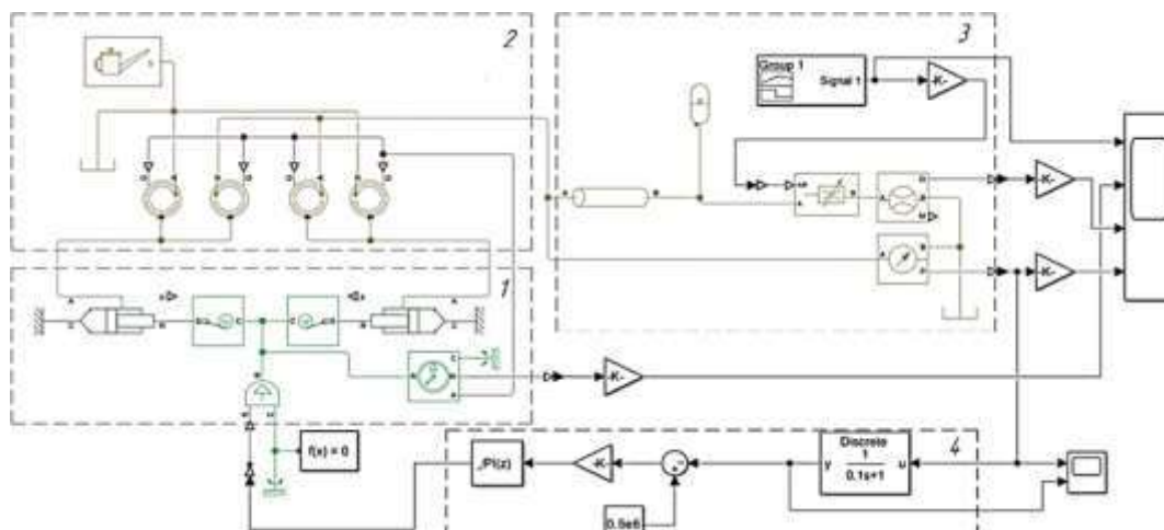
Рисунок 1 – Компьютерная модель системы подачи воды пароплазменной горелки Figure 1 – Computer model of the water pump displacement system for a steam plasma burner
