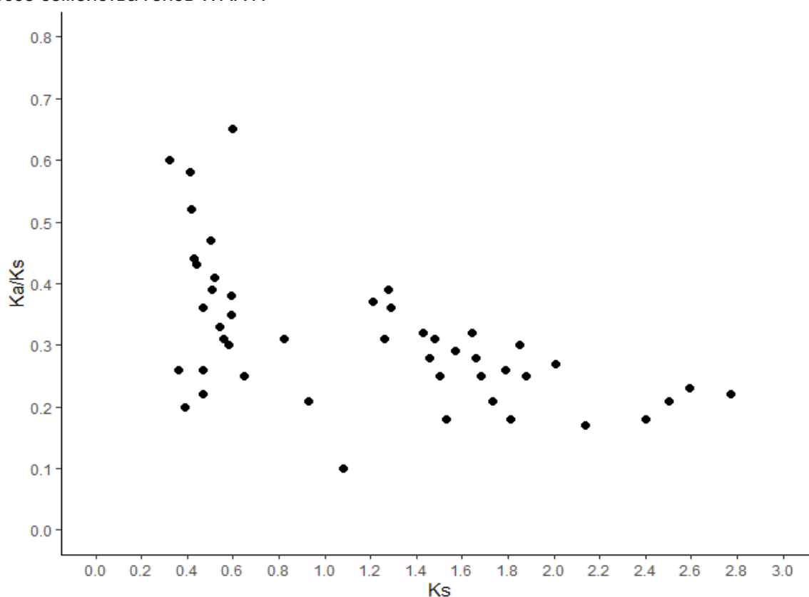
Рисунок 2 – Точечная диаграмма распределения Ka/Ks относительно Ks для выявленных дублированных генов RpWRKY . Каждая точка на диаграмме соответствует одной паре дублированных генов RpWRKY
