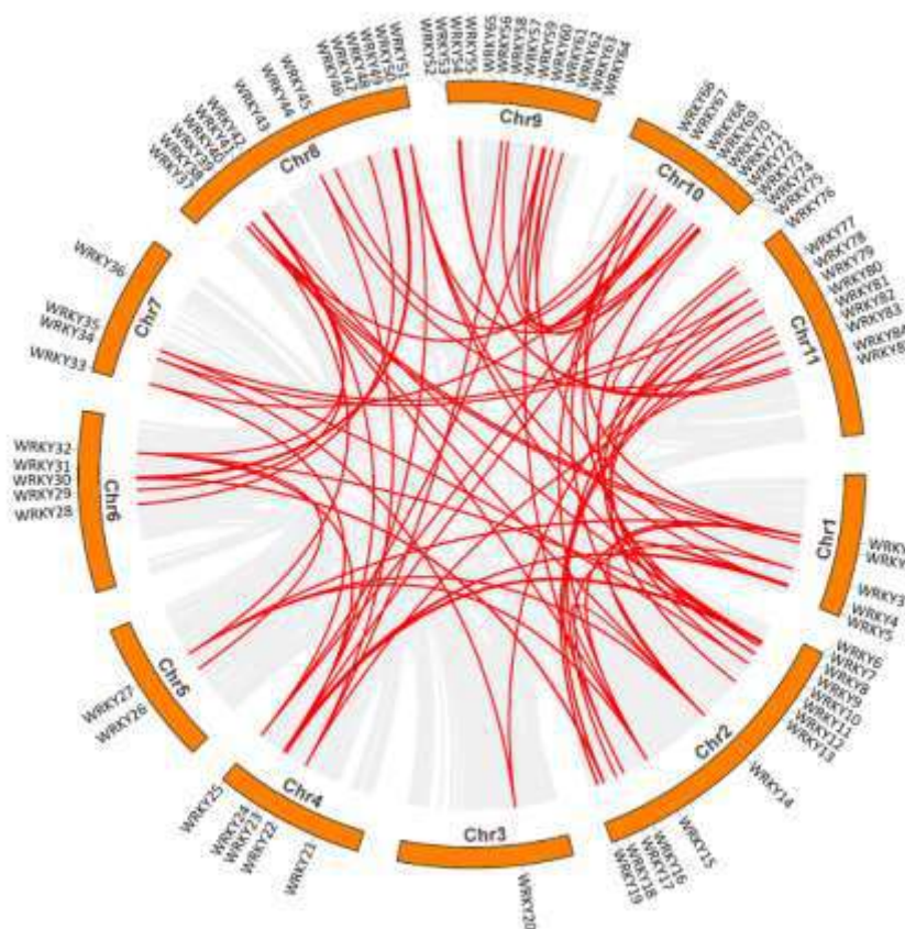
Рисунок 1 – Хромосомное расположение и дублицированные пары генов семейства транскрипционных факторов WRKY в геноме Robinia pseudoacacia . Коллинеарные (синтеничные) пары генов RpWRKY соединены красными линиями. Серые линии обозначают все остальные коллинеарные блоки, выявленные в геноме R. pseudoacacia
