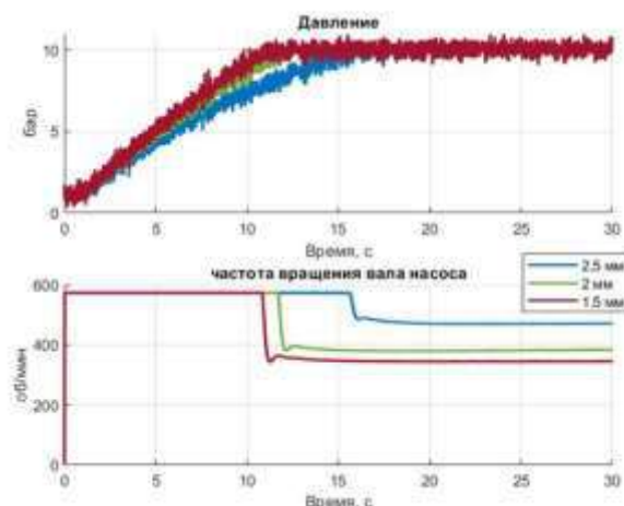
Рисунок 8 – Зависимости давления и частоты вращения вала насоса от времени при разном проходном сечении сопла форсунки при уставке давления 10 бар Figure 8 – The dependence of the pressure and speed of rotation of the pump shaft on time at different flow sections of the injector nozzle at a pressure setpoint of 10 bar
