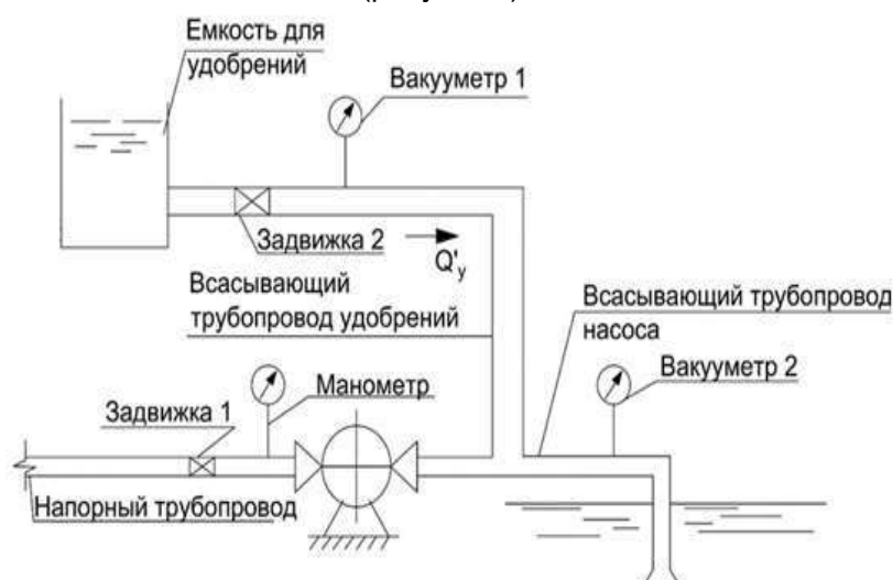
Рисунок 3 – Схема ввода удобрений энергией всасывающего трубопровода насосной станции ООО «Рассвет» Куйбышевского района Ростовской области Figure 3 – Scheme of fertilizer input using the suction pipeline of the pumping station of LLC «Rassvet» in the Kuibyshevsky District of the Rostov Region
