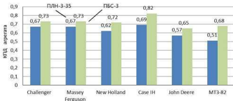
Рисунок 2 – Диаграмма КПД пахотных агрегатов с плугами ПЛН-3-35 и ПБС-3 Figure 2 – Efficiency diagram of ploughing units with PLN-3-35 and PBC-3 ploughs
