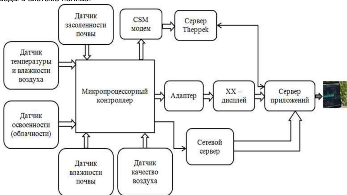
Рисунок 5 – Структурная схема автоматизации управления поливом с применением технологии «Интернета вещей»
