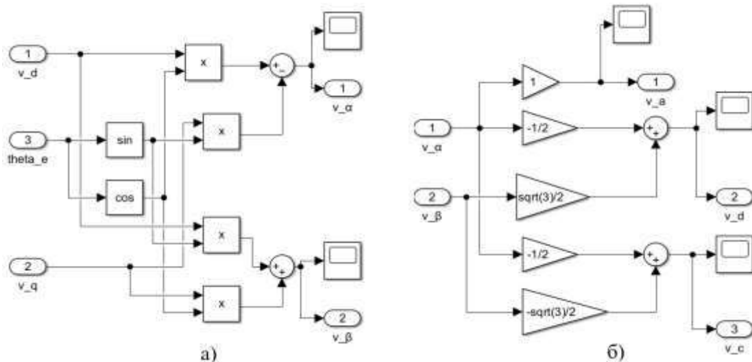
Рисунок 5 – Подсистемы перехода из вращающейся системы координат ( dq ) в неподвижную ( abc ): а) подсистема обратного преобразования Парка; б) подсистема обратного преобразования Кларка Figure 5 – Transition from a rotating system to a three-phase coordinate system: a) the subsystem of the inverse Park transformation; b) the subsystem of the inverse Clark transform
