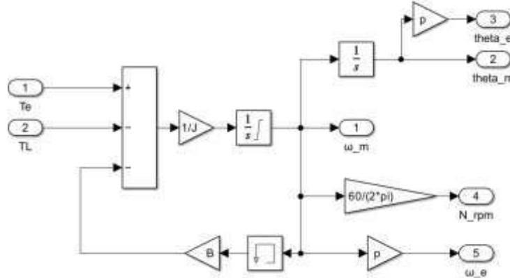
Рисунок 3 – Механическая подсистема Figure 3 – Mechanical subsystem
