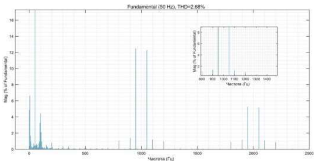
Рисунок 8 – Спектр фазного тока при векторном управлении (THD = 2,68 %)
