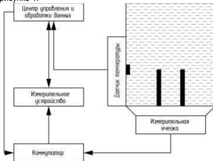
Рисунок 1 – Структура измерительно-аналитической установки Figure 1 – Structure of the measuring and analytical installation
