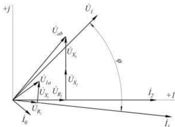
Рисунок 3 – Векторная диаграмма токов и напряжений ТВЧ индуктора с нагрузкой-теплообменником: \dot{I}_1 – комплекс тока в индукторе; \dot{I}_2 – комплекс тока в теплообменнике; \dot{I}_0 – комплекс тока в сопротивлении обратного замыкания; \dot{U}_{R1} и \dot{U}_{X1} – активная и реактивная составляющие комплекса напряжения на соответствующих сопротивлениях индуктора; \dot{U}_{R2} и \dot{U}_{X2} – активная и реактивная составляющие комплекса напряжения на соответствующих сопротивлениях теплообменника; \dot{U}_{1a} и \dot{U}_{1b} – комплексы напряжений между соответствующими узлами схемы замещения; \dot{U}_1 – комплекс напряжения на зажимах индуктора схемы замещения
