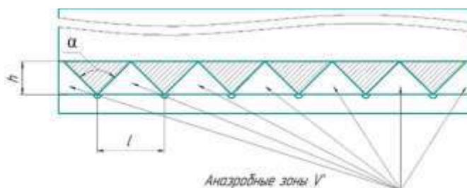
Рисунок 5 – Анаэробные зоны в камере установки Figure 5 – Anaerobic zones in the plant chamber
