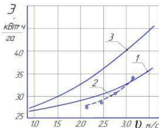
Рисунок 5 – Зависимость энергоемкости обработки почвы пахотными агрегатами МТЗ-82 + ПБС-3 и МТЗ-82 + ПЛН-3-35: 1 – теоретическая зависимость МТЗ-82 + ПБС-3; 2 – экспериментальная зависимость МТЗ-82 + ПБС-3; 3 – теоретическая зависимость МТЗ-82 + ПЛН-3-35
