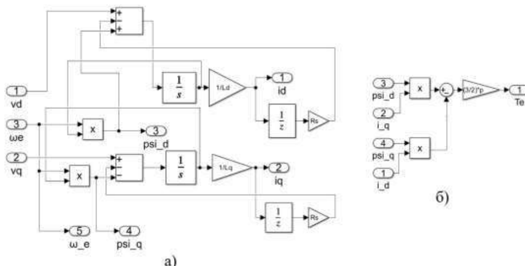
Рисунок 2 – Математическая модель СРД в осях dq : а) подсистема уравнений напряжения в осях dq ; б) подсистема расчёта электромагнитного момента Figure 2 – Mathematical model of SynRM in the dq axes: а) subsystem of stress equations in the dq axes; б) subsystem for calculating the electromagnetic moment
