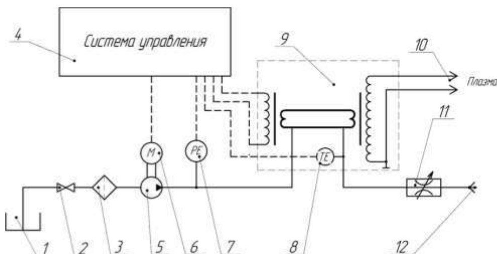
Рисунок 3 – Схема гидравлической системы пароплазменной жидкотопливной горелки.
