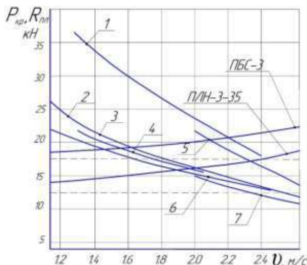
Рисунок 1 – Зависимость тягового усилия P_{кр} тракторов (1 – Case IH JX1090U; 2 – Massey Ferguson 4325; 3 – Challenger MT 425; 4 – John Deere 5085; 5 – New Holland TD5030; 6 – MT3-82; 7 – MTZ-80) и тягового сопротивления плуга R_{пл} от скорости движения u_p (пунктиром отмечен диапазон силы тяги трактора в тяговом классе 1,4)
