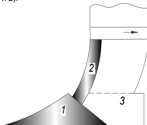
Рисунок 1 – Лемех плуга Figure 1 – Ploughshare
