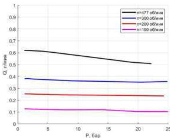
Рисунок 5 – Зависимости подачи от давления радиально-плунжерного насоса Figure 5 – Dependence of pump displacement on the pressure of a radial plunger pump
