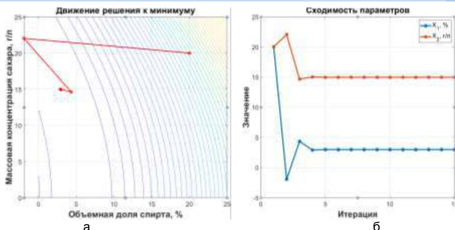
Рисунок 5 – Контурная карта функции невязки (а) и график сходимости параметров (б) при X_1 = 3\% и X_2 = 15 г/л
