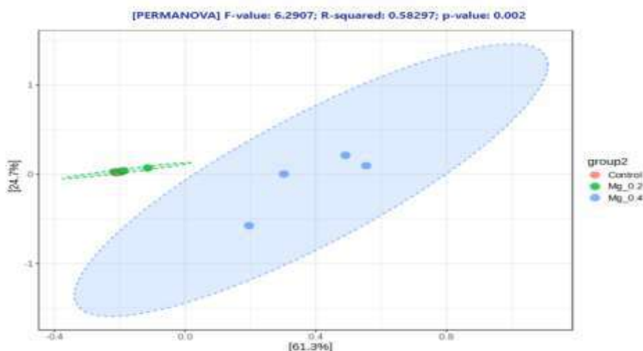
Рисунок 4 – 2D диаграмма ординации кишечной микробиоты рыб контрольной и опытных групп, построенная методом главных координат на основе дистанций Брея-Кёртиса (опытные группы: Mg_0.2 и Mg_0.4 – добавка ультрадисперсных частиц магния в концентрациях 0,2 и 0,4 ppm; Control – контрольная группа)
