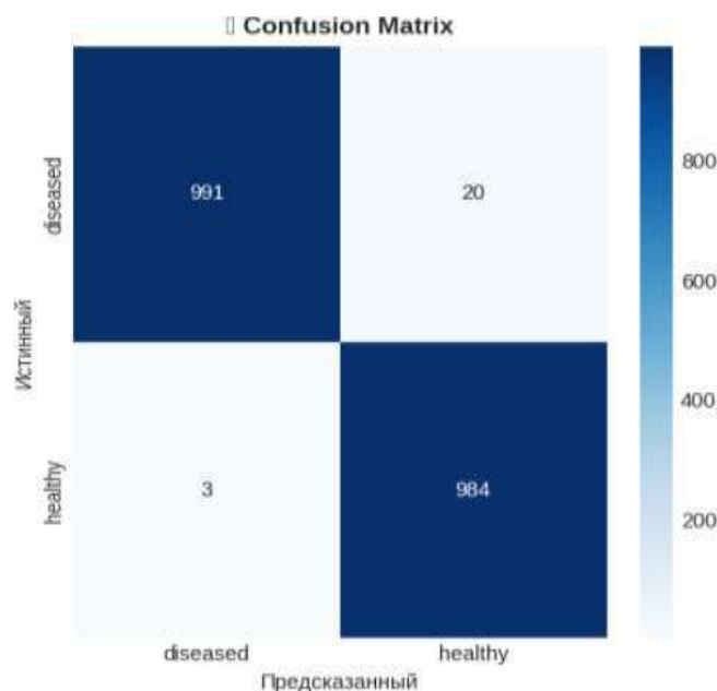
Рисунок 6 – Матрица ошибок (confusion matrix) разработанной нейронной сети на валидационной выборке из 1 998 изображений (составлено авторами)
