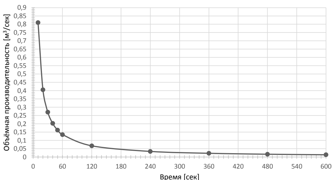
Рисунок 3 – Зависимость объёмной производительности насоса от времени необходимого для проведения всего процесса охлаждения
