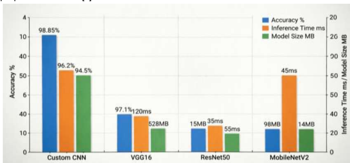
Рисунок 2 – Сравнительный анализ производительности различных архитектур сверточных нейронных сетей для задач классификации плодов яблоки (Custom CCN-созданная авторами)
