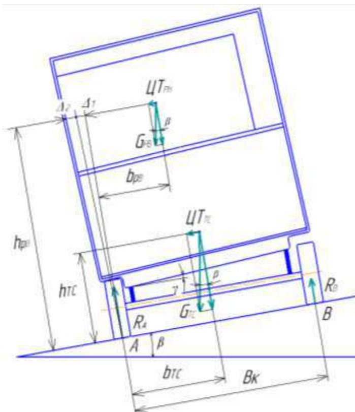
Рисунок 3 – Схема сил, действующих на ПТРС-2 при его движении в поперечном к уклону направлении
