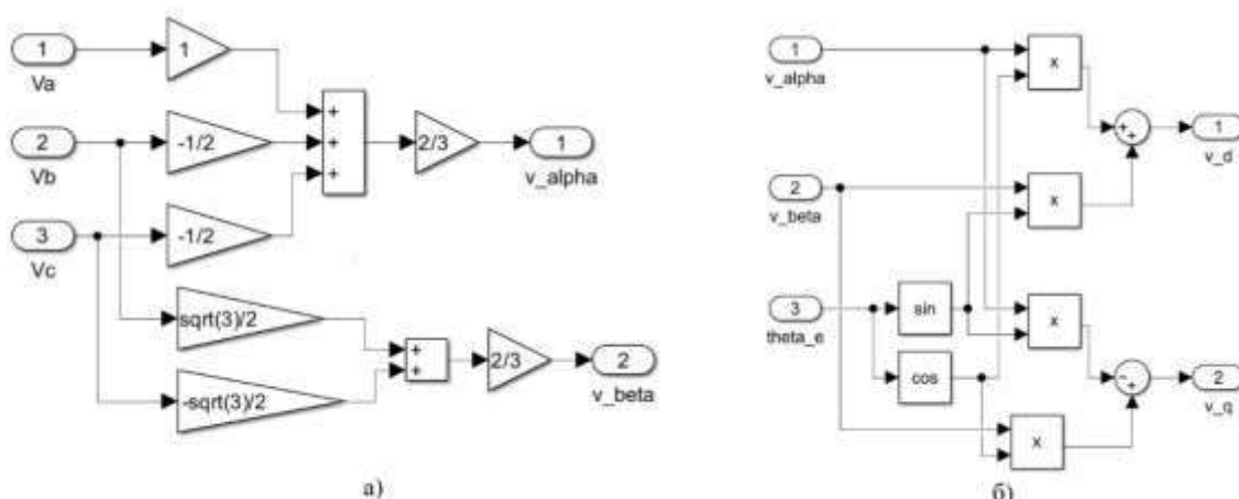
Рисунок 1 – Переход из трёхфазной системы координат во вращающуюся систему dq :
