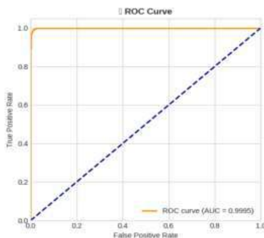
Рисунок 5 – ROC-кривая разработанной сверточной нейронной сети (составлено авторами)
