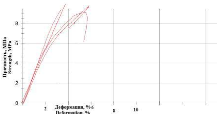
Рисунок 7 – График зависимости деформации от прочности образца 4 с содержанием кукурузной мезги в количестве 10,52 %, пектина – 2,98 %, глицерина – 2,19 %, кальция – 1,05 % и формовки методом горячего прессования
