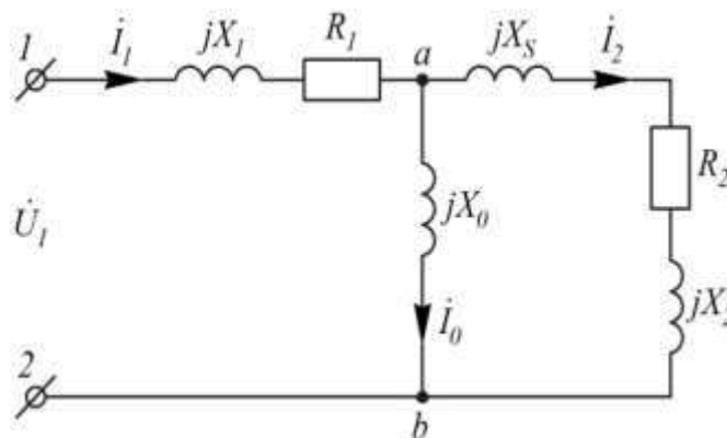
Рисунок 2 – Расчетная электрическая эквивалентная схема замещения индуктора с загрузкой-теплообменником: R_1, jX_{M1} – активное и индуктивное сопротивления индуктора, Ом; R_2, jX_{M2} – активное и индуктивное сопротивления теплообменника, Ом; jX_S – индуктивное сопротивление рассеяния, Ом; jX_0 – индуктивное сопротивление обратного замыкания, Ом; \dot{U}_1 – комплекс напряжения на индукторе с загрузкой, В; \dot{I}_1 – комплекс тока в индукторе, А; \dot{I}_2 – комплекс тока в нагрузке индуктора, А; \dot{I}_0 – комплекс тока в реактивном сопротивлении обратного замыкания, А
