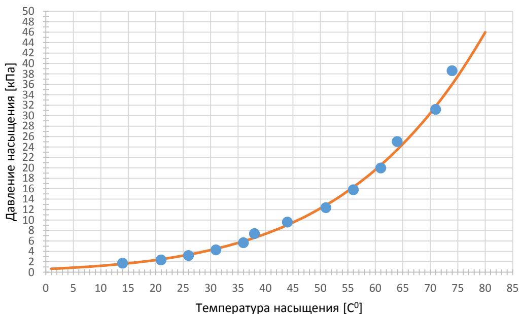
Рисунок 4 – Экспериментально полученная зависимость температуры насыщения воды от давления
