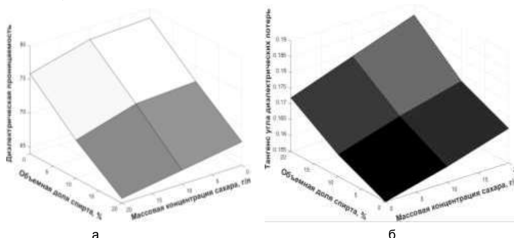
Рисунок 2 – Зависимость диэлектрической проницаемости (а) и тангенса угла потерь (б) от объемной доли спирта и массовой концентрации сахара в растворе
