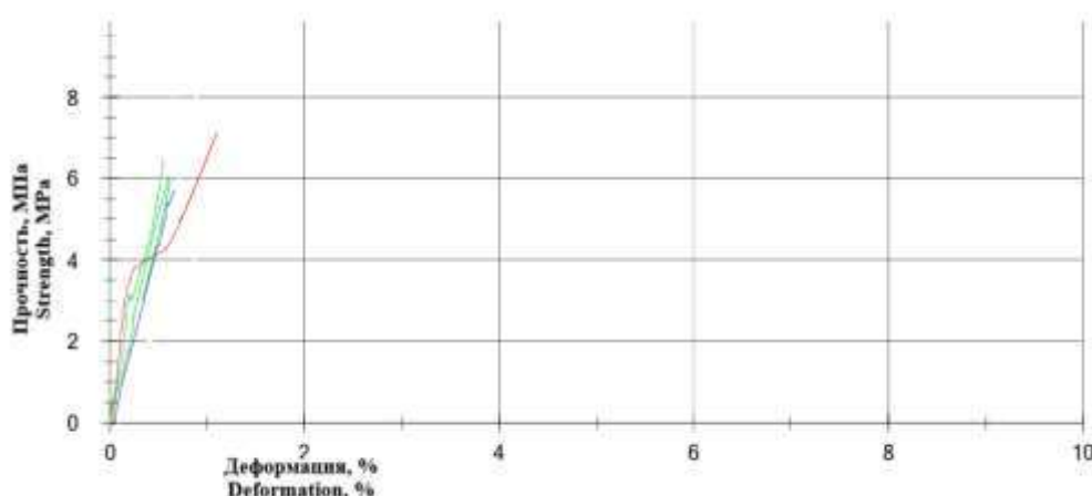
Рисунок 5 – График зависимости деформации от прочности образца 3 с содержанием кукурузной мезги в количестве 10,6 %, пектина – 3,00 %, глицерина – 2,2 % и формовки методом горячего прессования Figure 5 – Stress-strain curve for a sample 3 containing 10.6 % corn pulp, 3.00 % pectin, 2.2 % glycerol, and formed by the hot pressing method
