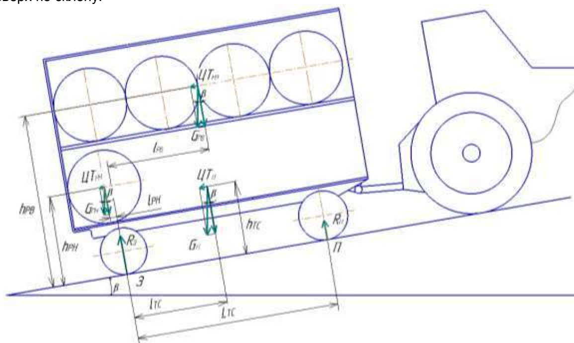
Рисунок 5 – Схема сил, действующих на ПТРС-2 при его движении в продольном к склону направлении Figure 5 – Diagram of forces acting on the loading vehicle-2 during its movement in the direction of the slope
