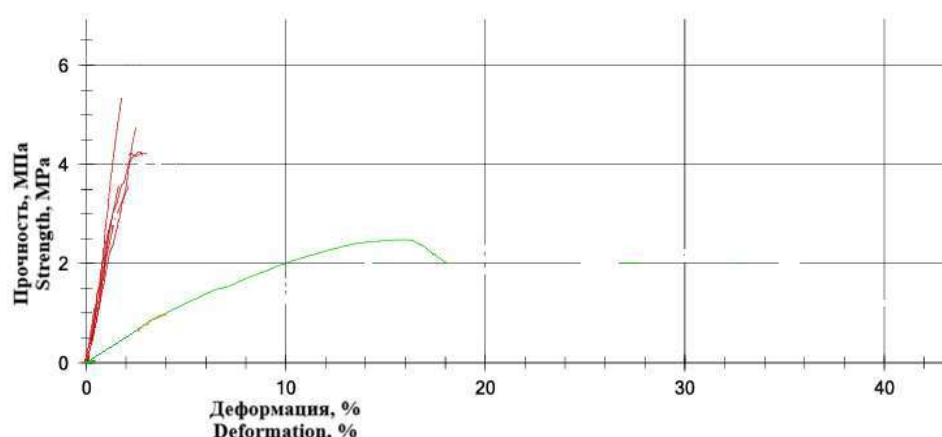
Рисунок 3 – График зависимости деформации от прочности образца 2 с содержанием кукурузной мезги в количестве 10,3 %, пектина – 3,00 %, глицерина – 2,21 % и формовки методом раскатки Figure 3 – Deformation versus strength graph for a sample 2 with a composition of 10,3 % corn bran, 3,00 % pectin, 2,21 % glycerol, molded using the rolling method
