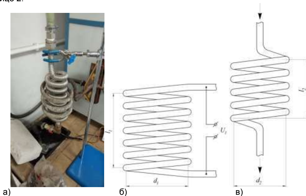
Рисунок 1 – Индукционный нагреватель молока токами высокой частоты (ТВЧ): а) – общий вид нагревательной установки; б) – геометрические параметры цилиндрического многovitкового индуктора; в) – геометрические параметры змеевикового теплообменника, где d_1 – диаметр цилиндрического многovitкового индуктора, d_1=0,1 м; l_1 – длина индуктора, l_1=0,3 м; d_2 – диаметр змеевикового теплообменника, d_2=0,08 м; l_2 – длина теплообменника, l_2=0,225 м
