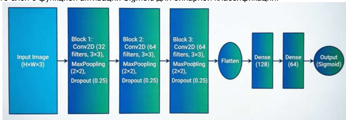
Рисунок 3 – Архитектура разработанной нейронной сети со сверточными слоями для классификации плодов яблоки (составлено авторами)
