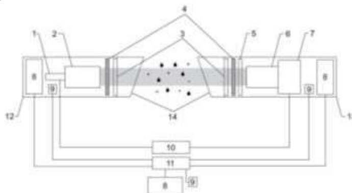
Рисунок 2 – Устройство голографического дистрометра
