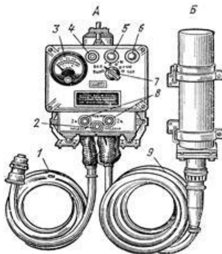
Рисунок 2 – Рентгенометр ДП-3Б
