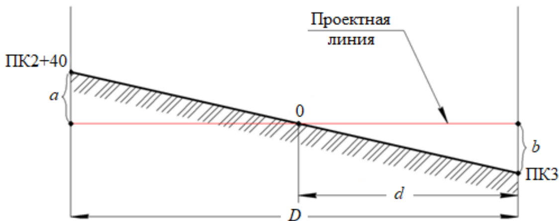
Рисунок 8 – Определение расстояний от точки нулевых работ до связующих точек
