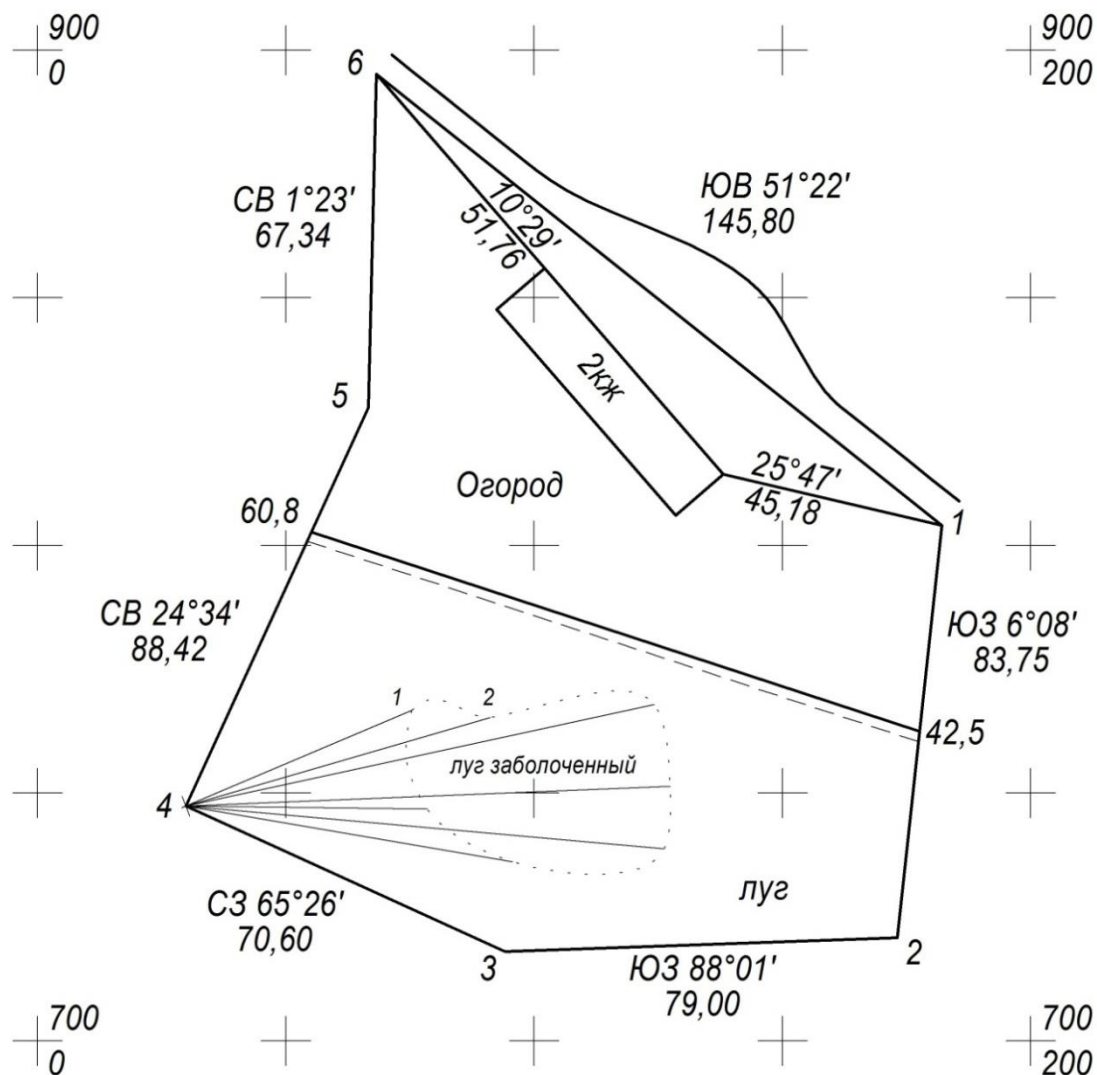
Рисунок 3 – Абрис теодолитной съёмки
