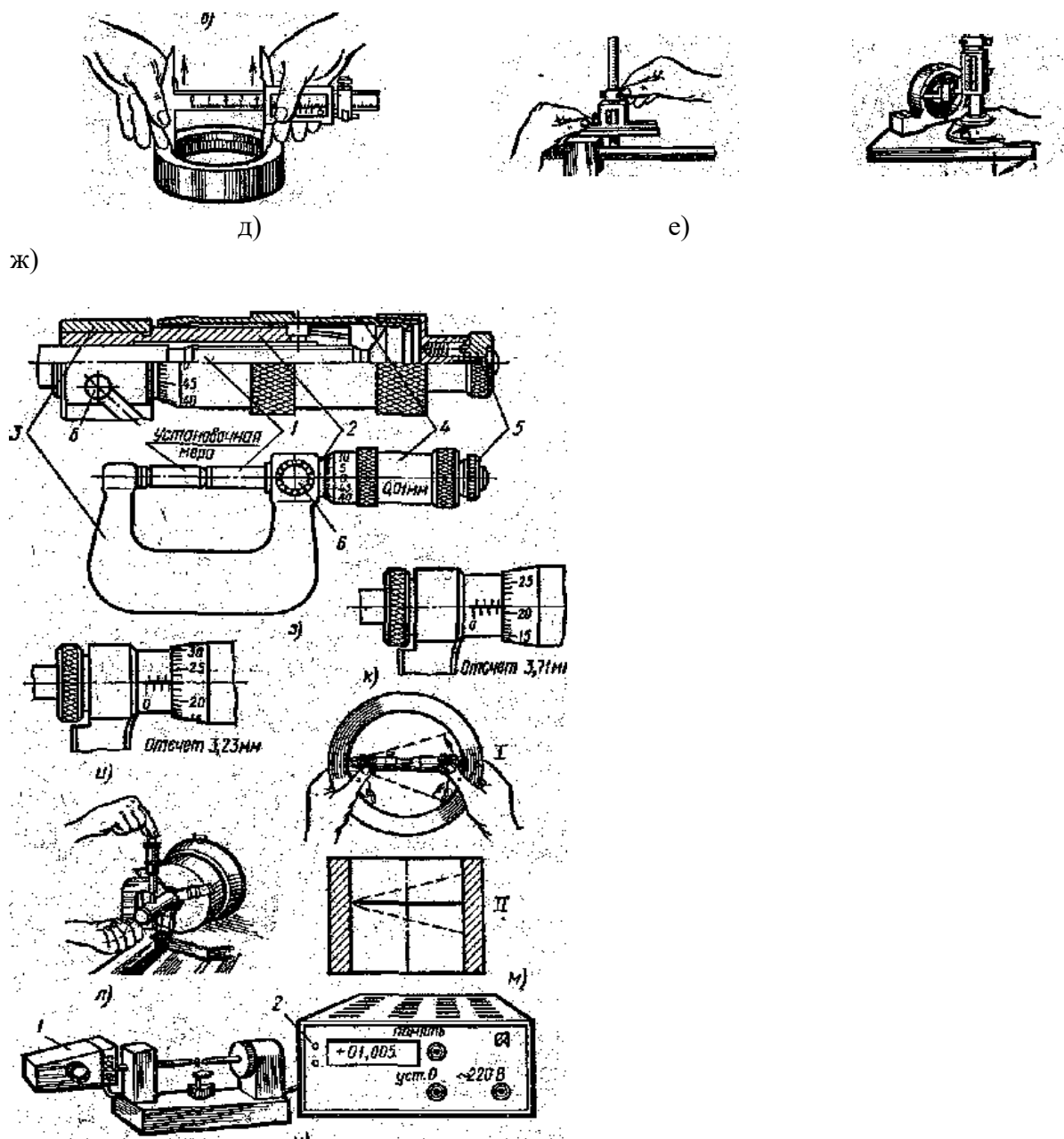
Рис.2. Штангенприборы микрометрические приборы:
