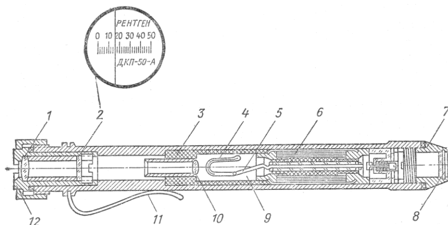
Рисунок 11 - Дозиметр ДКП-50А
