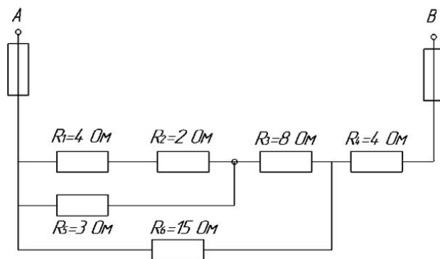
Рисунок 6 – Электрическая схема
