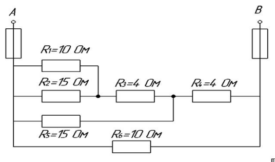
Рисунок 4 – Электрическая схема
