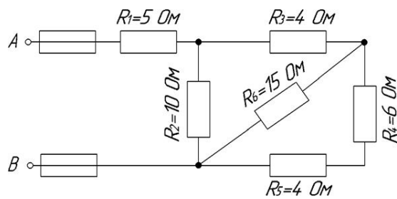
Рисунок 3 – Электрическая схема
