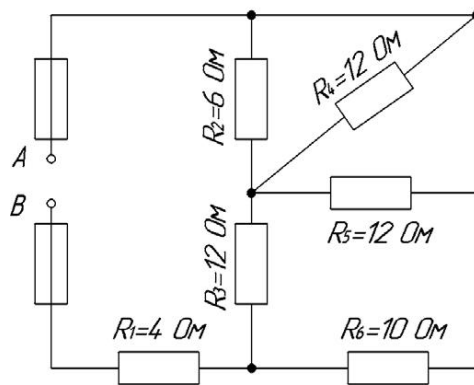
Рисунок 7 – Электрическая схема
