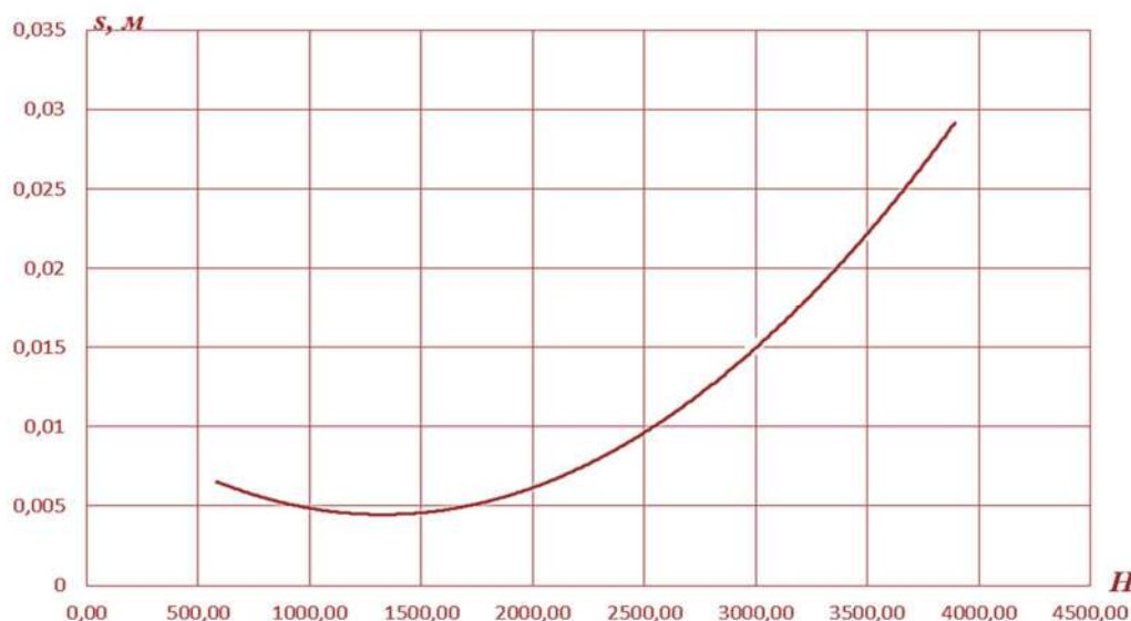
Рисунок 7 – Генерируемое усилие и перемещение носка рабочего органа
