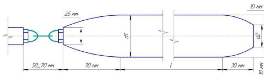
Рисунок 7 – Схема уширителя для кротователя №1 конусоцилиндрической формы
