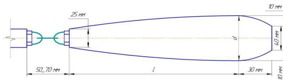
Рисунок 8 – Схема уширителя для кротователя № 2 конусопараболической формы
