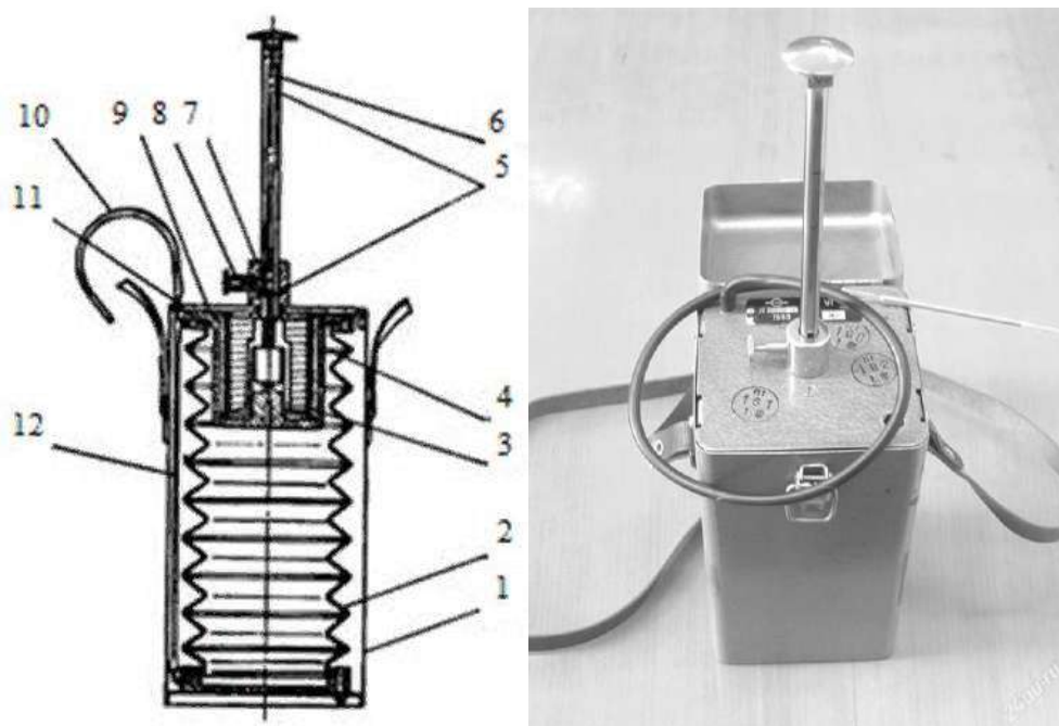
Рисунок 7 - Универсальный переносной газоанализатор УГ-2
