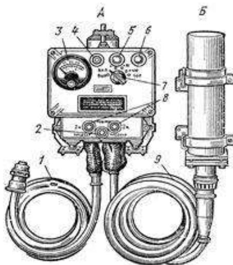
Рисунок 2 – Рентгенметр ДП-3Б
