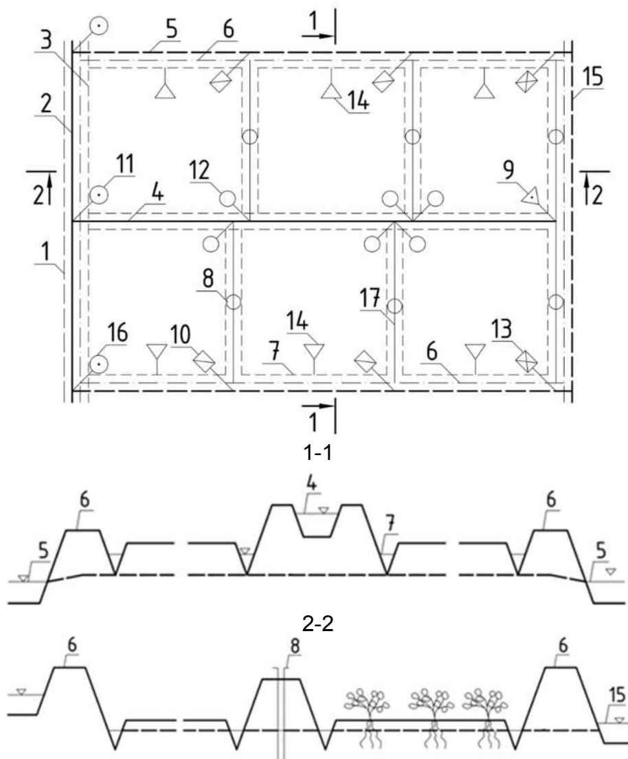
Рисунок 2 – Усовершенствованная карта-схема поливной карты Краснодарского типа:
