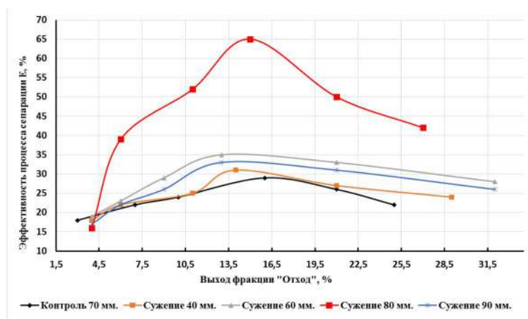
Рисунок 5 – График эффективности процесса сепарации отходов послеуборочной обработки сои при постоянной удельной зерновой нагрузке и разном соотношении выходов отходов Figure 5 – Graph of the efficiency of the post-harvest soybean waste separation process with a constant specific grain load and a different ratio of waste outputs
