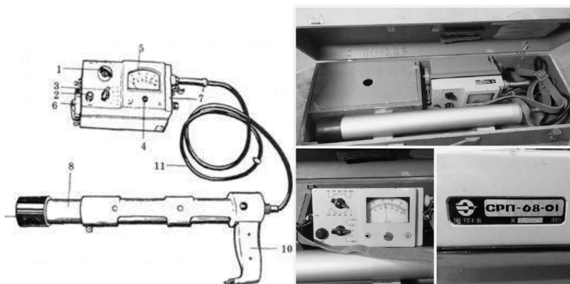
Рисунок 3 - Сцинтилляционный радиометрический прибор СПР -68-01
