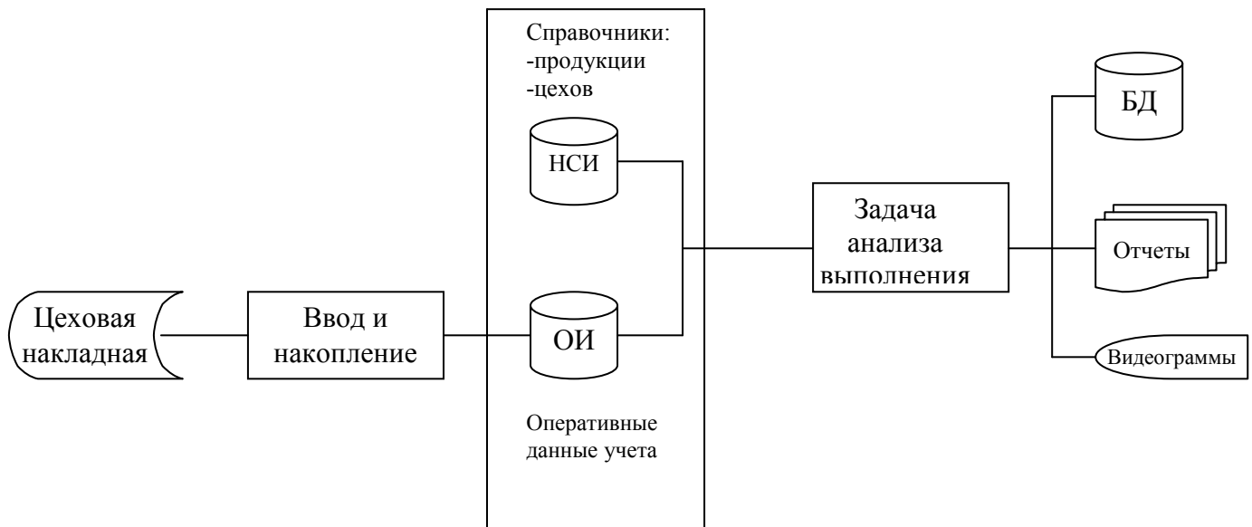
Схема решения задачи анализа выполнения плана
