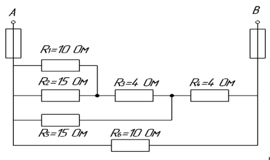
Рисунок 4 – Электрическая схема
