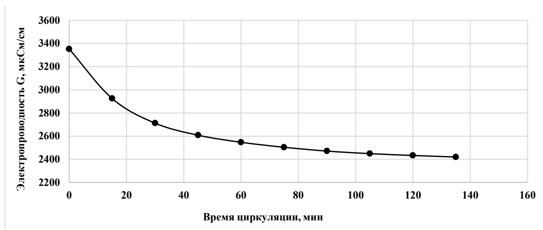
Рисунок 2 – Зависимость электропроводности раствора карбоната кальция от времени циркуляции в турбулентном режиме при скорости воды 0,5 м/с под воздействием электромагнитных волн прибора Термит
