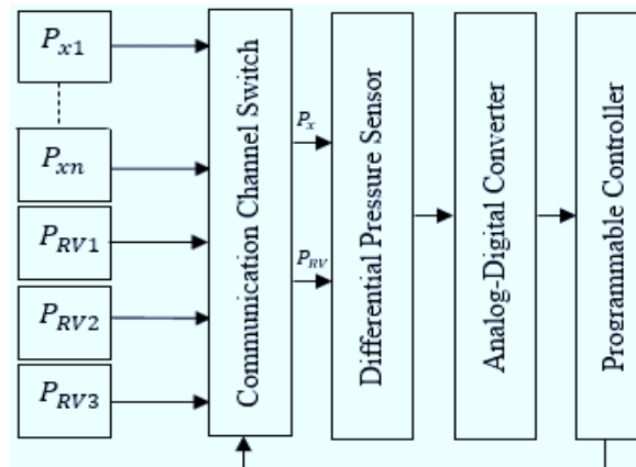
Figure 3 – IMS structure with three sample signals Рисунок 3 – Структура IMS с тремя сигналами выборки
