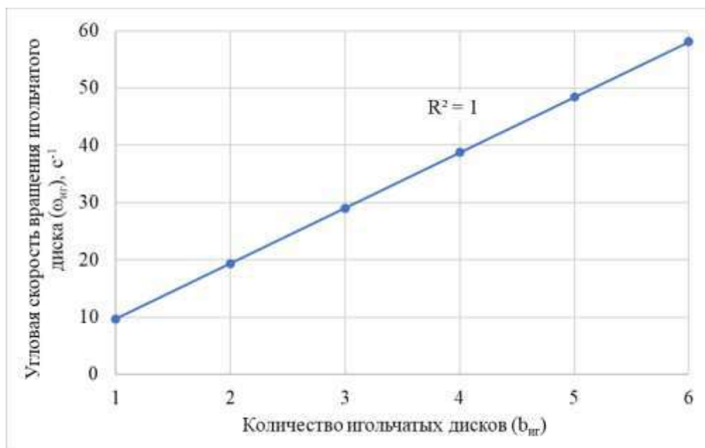
Рисунок 2 – График зависимости угловой скорости вращения ИД от их количества Figure 2 – Graph of the dependence of the angular velocity of rotation of the needle disk on their number
