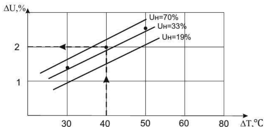
Рисунок 7 – Зависимость величины влагосъема с выжимки при сбросе давления от разности температур в сушильной камере и конденсаторе
