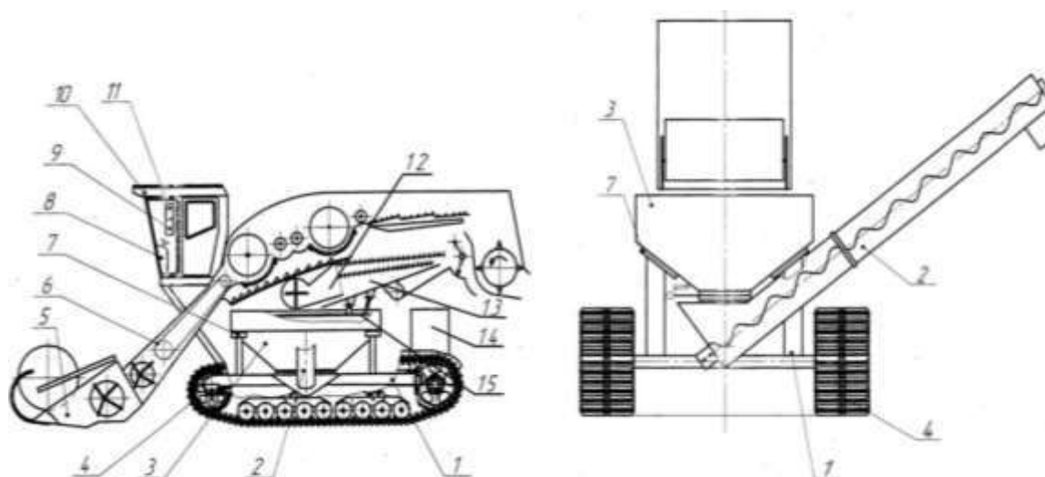
Рисунок 2 – Комбайн самоходный гусеничный зерноуборочный новой компоновки [19]:
