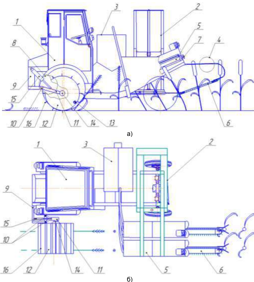
Рисунок 3 – Схема соргоуборочного комбайна: а) – вид сбоку; б) – вид сверху Figure 3 – Diagram of a sorghum harvester: a) side view; b) top view
