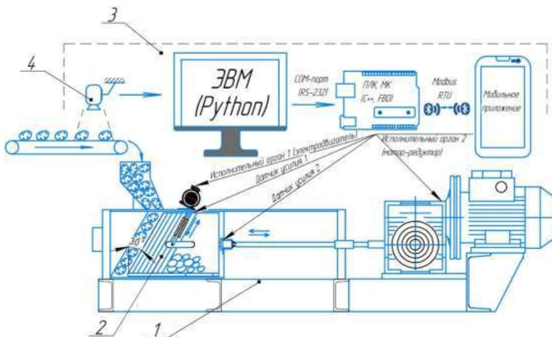
Рисунок 1 – Схема системы управления процессом комбинированного резания измельчителем корнеклубнеплодов: 1 – измельчитель корнеклубнеплодов; 2 – ножевая стенка; 3 – система управления; 4 – цифровая камера
