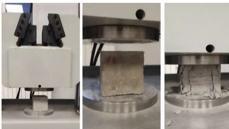
Рисунок 6 – Испытания образцов кубов на МИИ-100 Figure 6 – Compression testing of concrete cube specimens on the MII-100 machine
