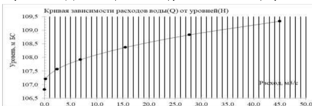
Рисунок 4 – График связи расхода с уровнями в НК Q=f(H) в створе после сооружения № 3 Figure 4 – graph of the relationship between flow rate and levels in the NK Q=f(H) in the section after structure No. 3
