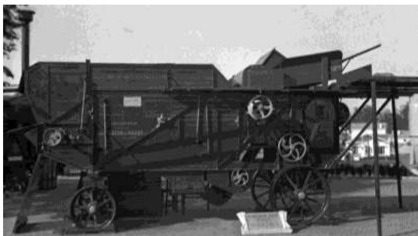
Фото 3 – Передвижная воздушно-решетчатая машина ВИМ-СМ-1 с ручной загрузкой Photo 3 – Mobile air-cleaner VIM-SM-1 with manual loading
