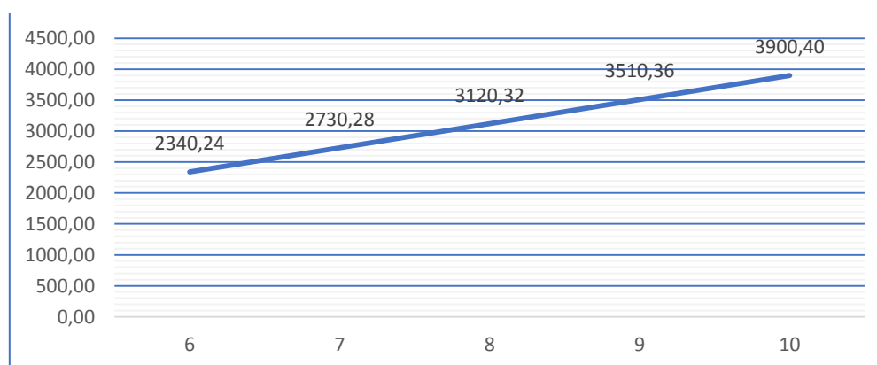
График 1 – Зависимость пружинящего усилия от толщины стенки трубы Graph 1 – Dependence of spring force on pipe wall thickness
