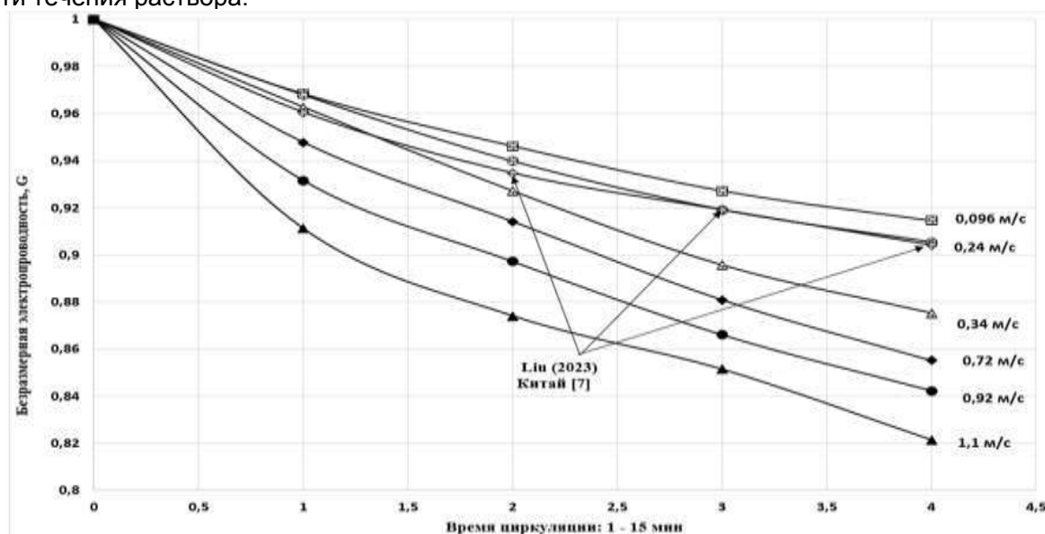
Рисунок 3 – Зависимость безразмерной электропроводности раствора \text{CaCO}_3 от времени циркуляции под воздействием ЭМП прибора Термит при различных скоростях течения раствора
