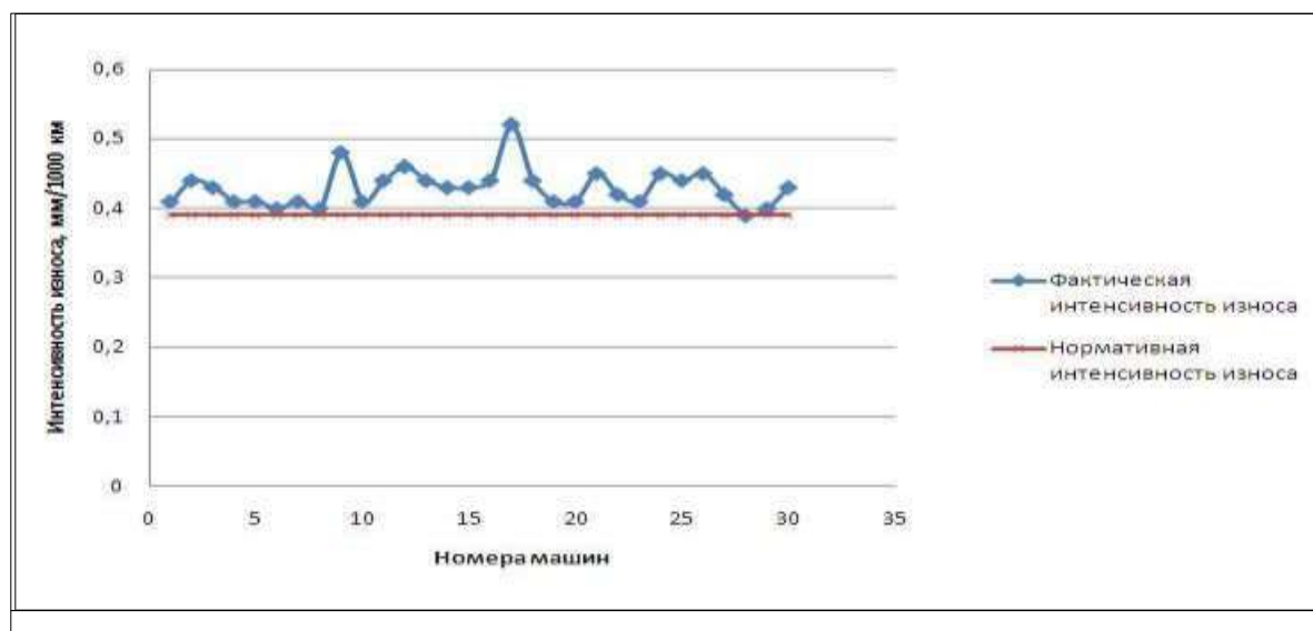
Рисунок 1 – График интенсивности износа исследуемых автомобильных шин марки ИД-П284 Figure 1 – Graph of wear intensity of the studied ID-P284 brand automobile tires
