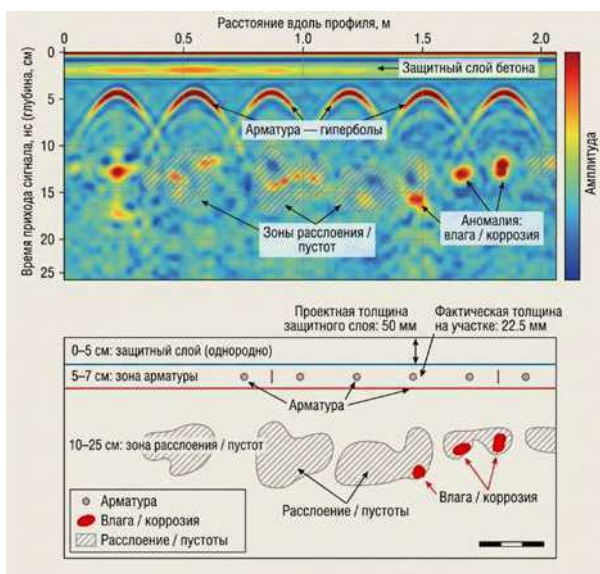
Рисунок 5 – Георадарный профиль бетонной конструкций ОС с дефектом Figure 5 – Ground-penetrating radar (GPR) profile of a concrete structure in the irrigation system showing a defect
