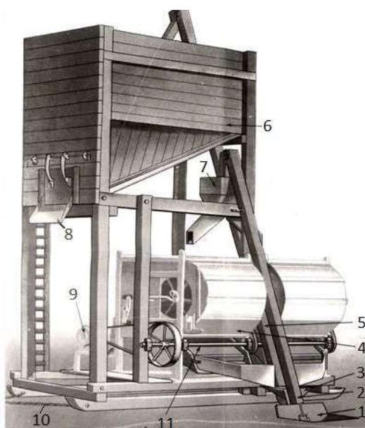
Фото 4 – Двухвеялочный зерноочистительный агрегат: 1 – завальная яма; 2 – транспортер; 3 – рама; 4 – веялка; 5 – транспортер; 6 – бункер; 7 – воронка; 8 – выпускной лоток; 9 – электродвигатель; 10 – прицеп; 11 – механический привод
