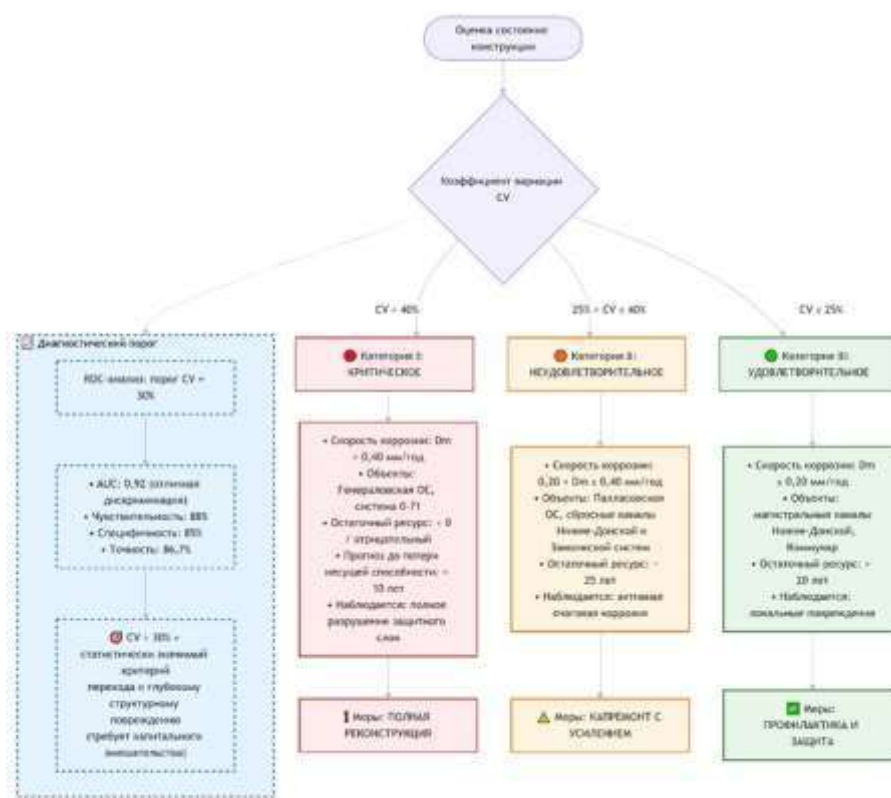
Рисунок 8 – Блок-схема оценки состояния ОС
