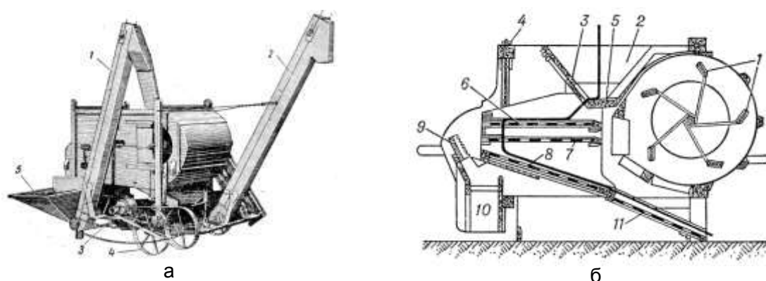
Рисунок 1 – Веялка-сортировка ВС-2,0 с транспортерами для зерна: а – общий вид; 1, 2 – элеваторы для зерна; 3 – электродвигатель; 4 – чугунные колеса; 5 – ковш; б – технологическая схема работы ВС-2,0: 1 – вентилятор; 2 – засыпной ковш; 3 – заслонка; 4 – регулятор наклона решет; 5 – колеблющееся дно ковша; 6, 7 и 8 – качающиеся проволочные решета; 9 – передвижной щиток; 10 – желоб для крупных примесей; 11 – неподвижное решето
