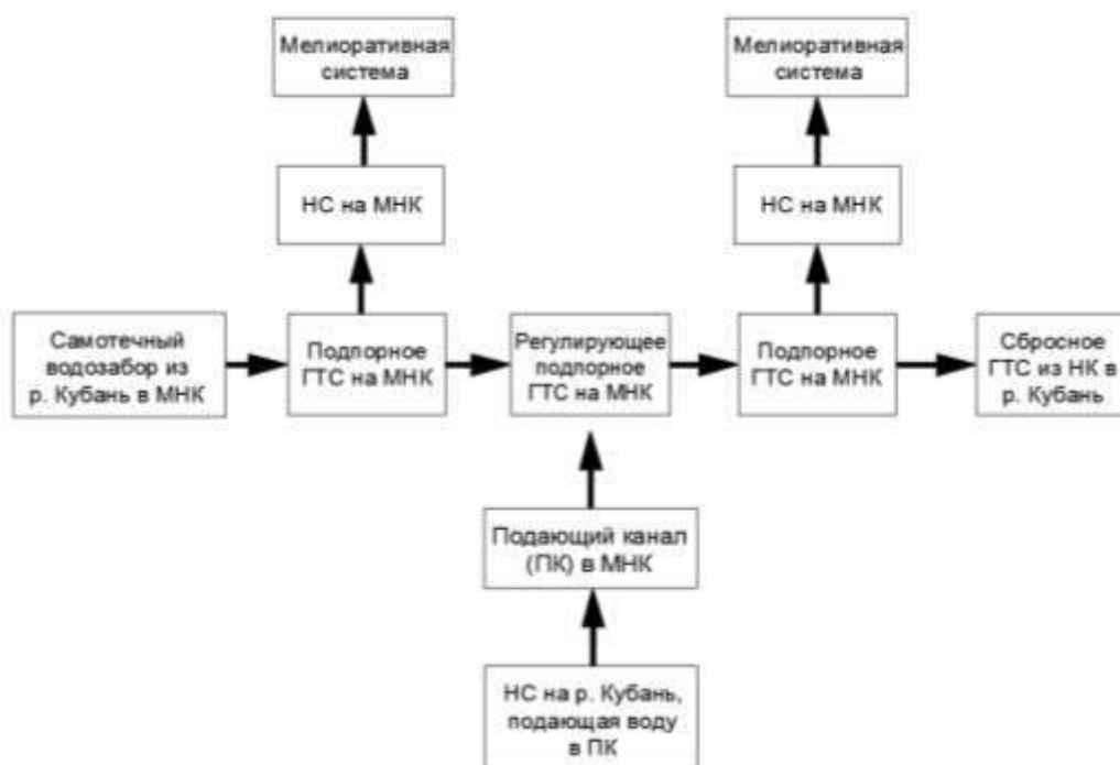
Рисунок 7 – Комбинированная схема водоподачи на мелиоративные системы Figure 7 – combined scheme of water supply to drainage systems
