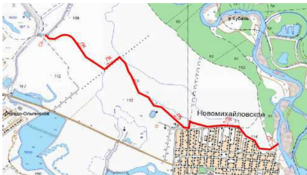
Рисунок 6 – Трасса для подачи дополнительного расхода подающим каналом из реки Кубань на мелиоративные системы Гулькевичского района
