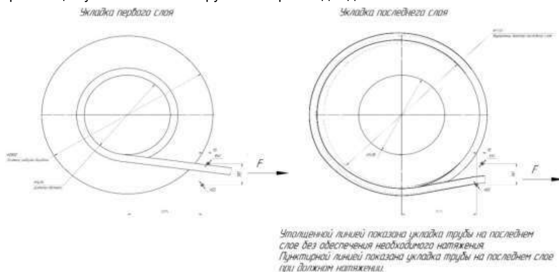
Рисунок 1 – Схема укладки трубы на барабан дождевальной машины
