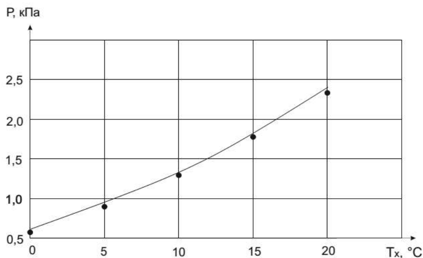
Рисунок 3 – Зависимость минимального остаточного давления в конденсаторе паров от температуры хладагента
