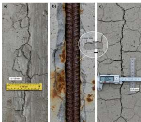
Рисунок 3 – Фотографии характерных дефектов бетонных конструкций мелиоративных сооружений Figure 3 – Photographs of characteristic defects in concrete structures of reclamation hydraulic facilities
