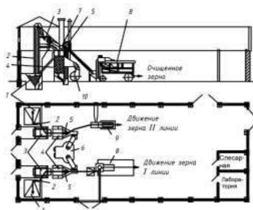
Рисунок 3 – Схема зерноочистительно-сушильного пункта: 1 – приемный бункер; 2, 5 – нории; 3 – веялка; 4 – зерносушилка; 6 – сушилка; 7 – механическая передача; 8, 9 – зерноочистительные машины; 10 – вентилятор сушилки
