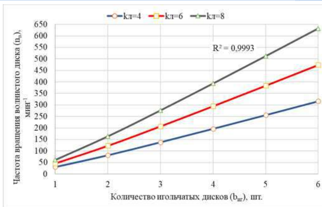
Рисунок 4 – Зависимость частоты вращения волнистых дисков от количества ИД Figure 4 – Dependence of the frequency of rotation of wavy discs on the number of needle discs
