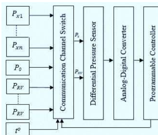
Figure 4 – The structure of the IMS with an iterative algorithm for correcting nonlinearity Рисунок 4 – Структура IMS с итеративным алгоритмом коррекции нелинейности
