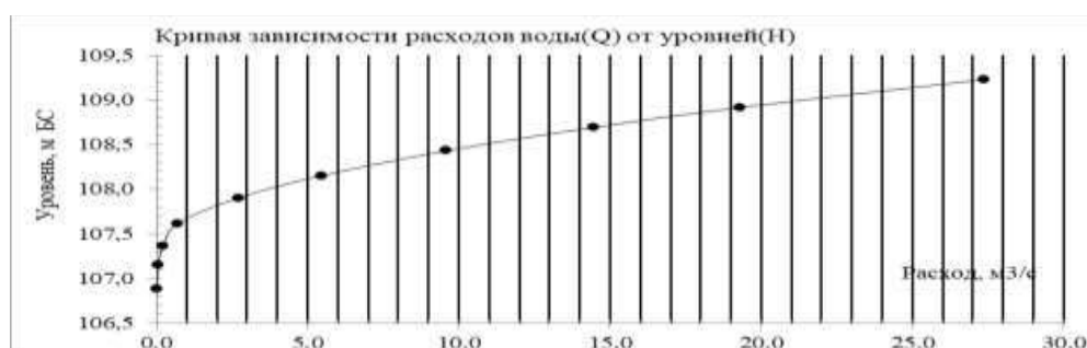
Рисунок 3 – График связи расхода с уровнями в МНК Q=f(H) в створе до сооружения № 3 Figure 3 – graph of the relationship between flow rate and levels in the MNC Q=f(H) in the section up to structure No. 3
