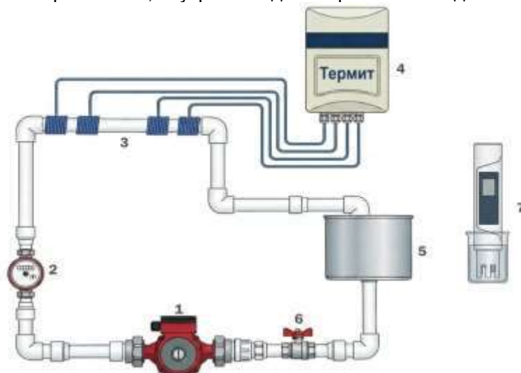
Рисунок 1 – Экспериментальная установка:
