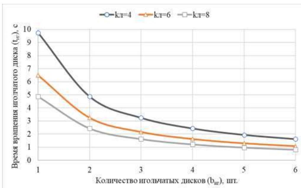
Рисунок 3 – График зависимости времени вращения ИД от их количества Figure 3 – Graph of the dependence of the rotation time of the needle disk on their number
