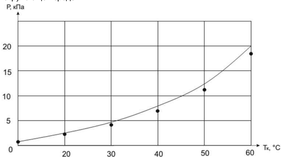
Рисунок 4 – Зависимость максимального остаточного давления в сушильной камере от температуры в калорифере
