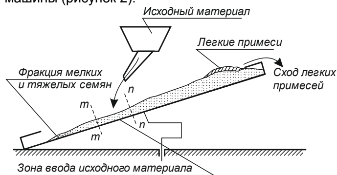
Рисунок 2 – Механическое кружало Figure 2 – Mechanical «kruzhalo»
