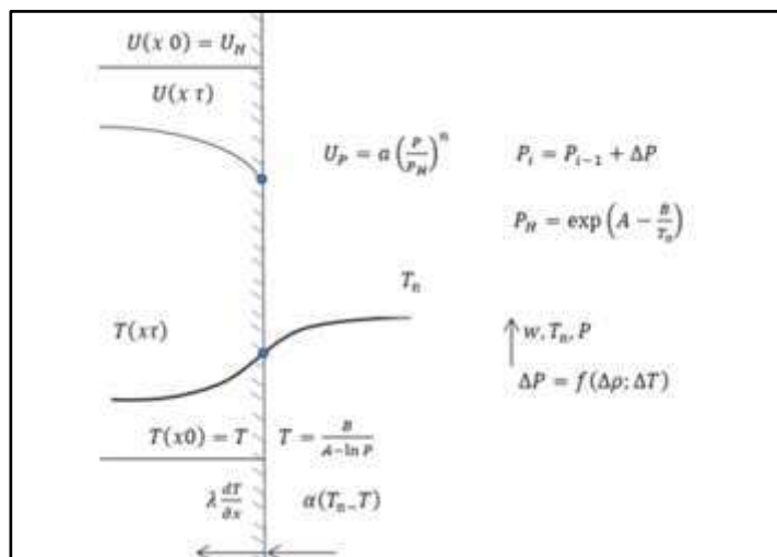
Рисунок 1 – Схема краевых условий при вакуум-осциллирующей сушке
