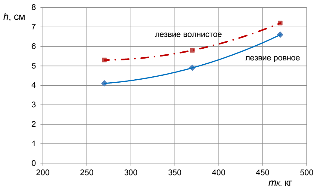
Рисунок 5 – Заглабление ножей катка в почву после измельчения растительных остатков зернового сорго
