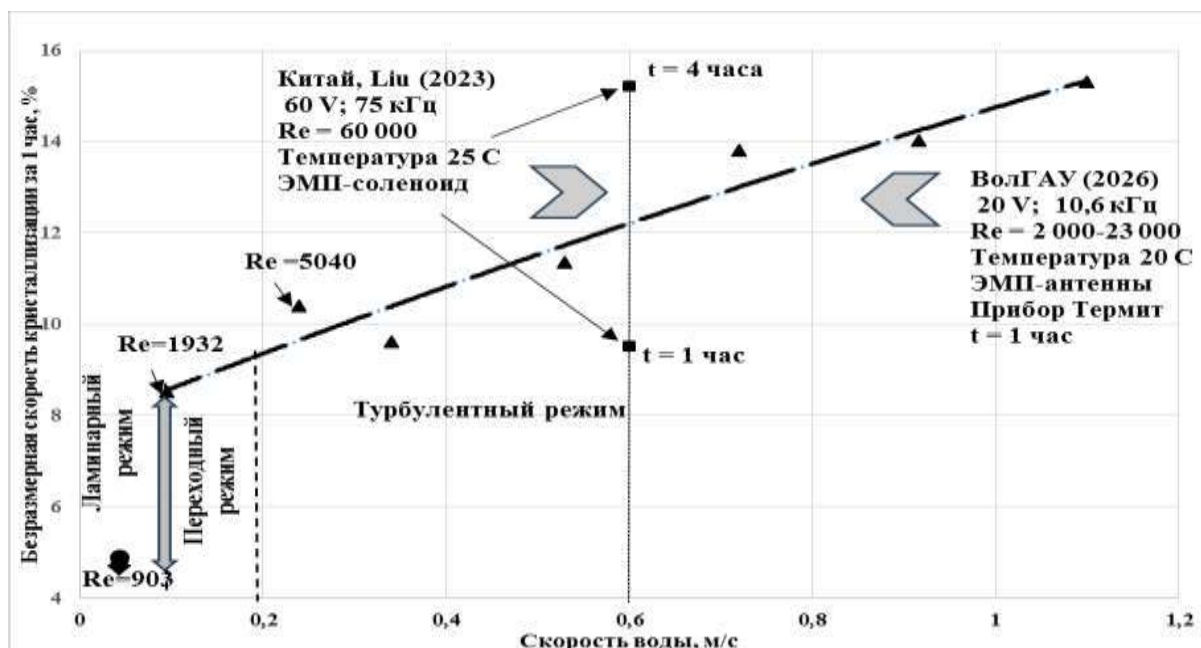
Рисунок 4 – Зависимость безразмерной скорости кристаллизации \text{CaCO}_3 от скорости течения раствора под воздействием электромагнитных волн прибора Термит
