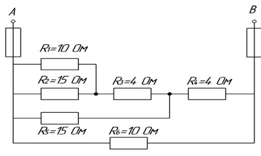
Рисунок 4 – Электрическая схема
