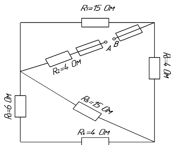
Рисунок 5 – Электрическая схема
