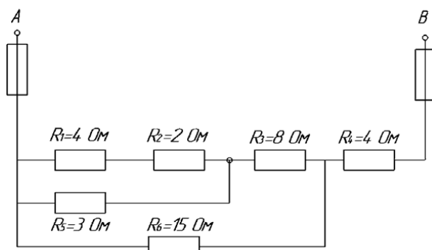
Рисунок 6 – Электрическая схема
