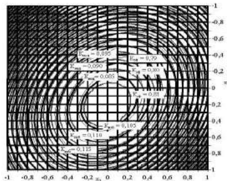
Рисунок 5 – Двумерное сечение для изучения влияния факторов диаметра насадка и расстояния между насадками при x_1 = -0,01 и x_3 = 0,02 на значения коэффициентов эффективного ( K_{эф} ), избыточного ( K_{изб} ) и недостаточного ( K_{нед} ) поливов
