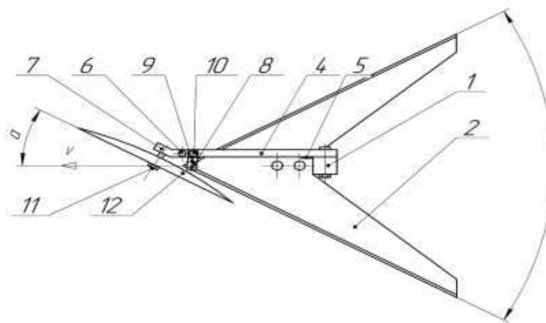
Рисунок 3 – Расположение сферического диска на стойке Figure 3 – Location of the spherical disk on the rack
