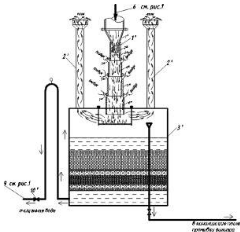
Рисунок 2 – Установка по очистке воды от взвесей, железа и др. примесей.
