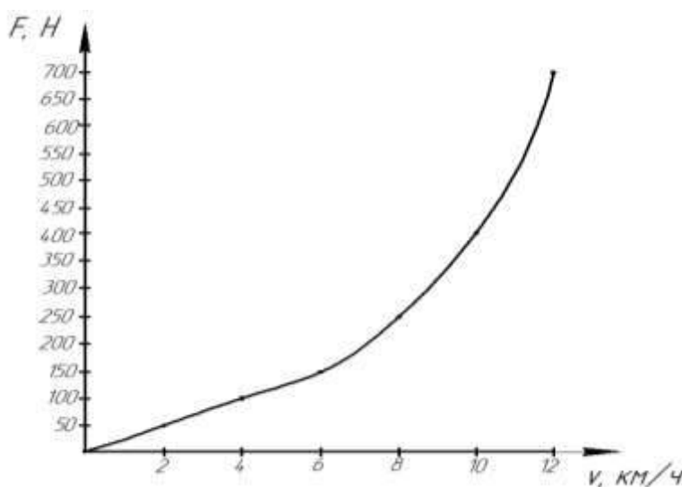
Рисунок 5 – Влияние скорости движения агрегата на тяговое сопротивление рабочего органа
