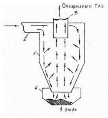
Рисунок 6.1. Схема возвратно-поточного циклона.
