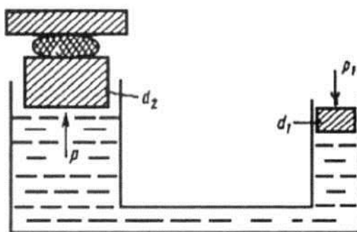
Рисунок 3.12 - Пресс гидравлический
