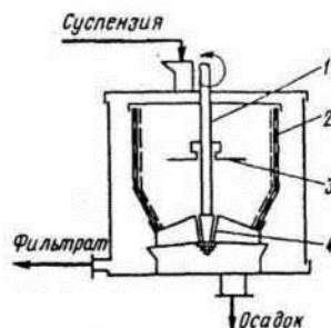
Рисунок 5.12 - Центрифуга с гравитационной выгрузкой осадка:
