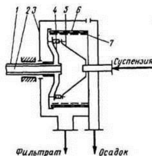
Рисунок 5.13 - Центрифуга непрерывного действия с пульсирующей выгрузкой осадка:
