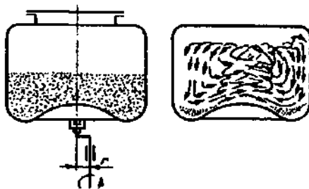
Рисунок 3.11. - Схема движения частиц в дражировочном грануляторе.
