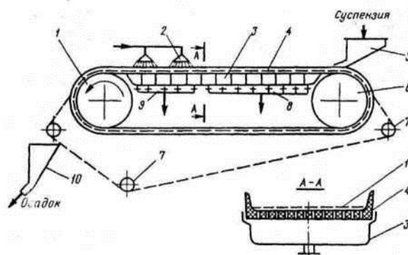
Рисунок 5.10 - Ленточный вакуум-фильтр:
