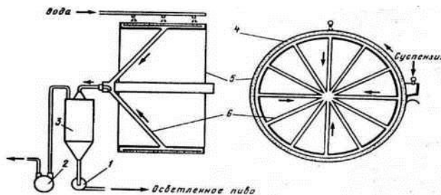
Рисунок 5.7 - Барабанный вакуум-фильтр:
