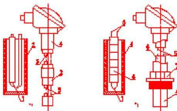
а - термопара ТПП; б - термопары ТХК и ТХА; 1 - рабочий спай; 2 - фарфоровый защитный чехол; 3 - фарфоровая трубка; 4 - металлическая трубка; 5 - термоэлектроды; 6 - фарфоровые бусы; 7 - неподвижный штуцер
