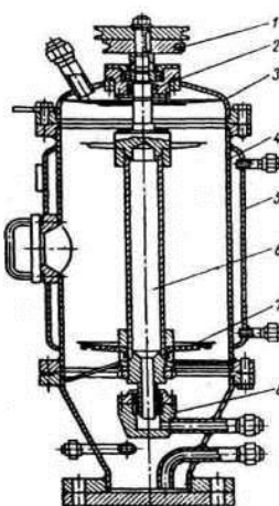
Рисунок 5.9 - Дисковый фильтр:
