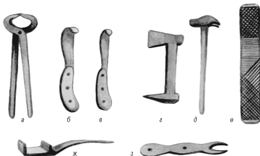
Рисунок 6. Ковочный инструмент: а – ковочные клещи; б – секач; в – обсечка; г – копытный нож; д – ковочный молоток; е – нашпиль; ж – лапа; з – шиповой ключ.
