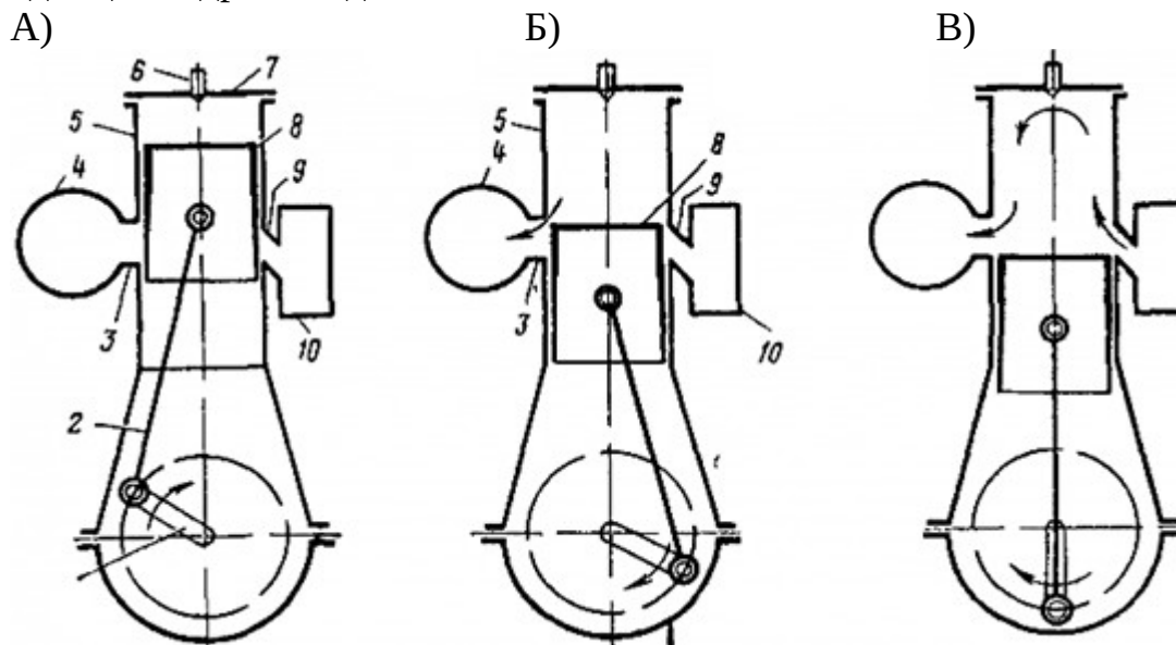
Рисунок 2.2 - Схема работы двухтактного дизеля
