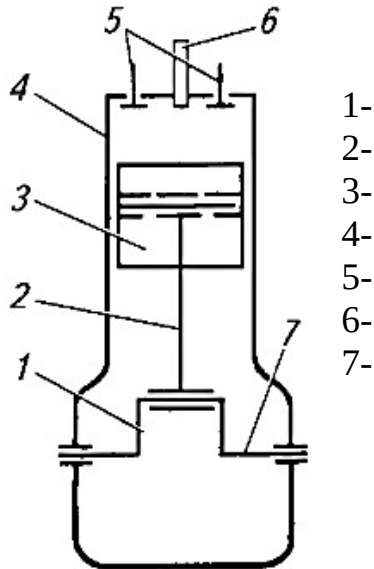
Рисунок 1 - Схема одноцилиндрового четырехтактного двигателя
