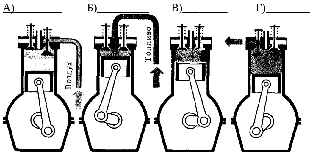
Рисунок 2.1 - Схема работы четырехтактного одноцилиндрового двигателя
