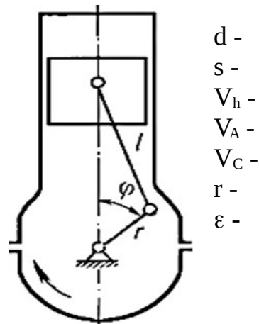
Рисунок 2 - Схема одноцилиндрового четырехтактного двигателя
