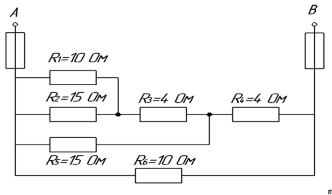
Рисунок 4 – Электрическая схема
