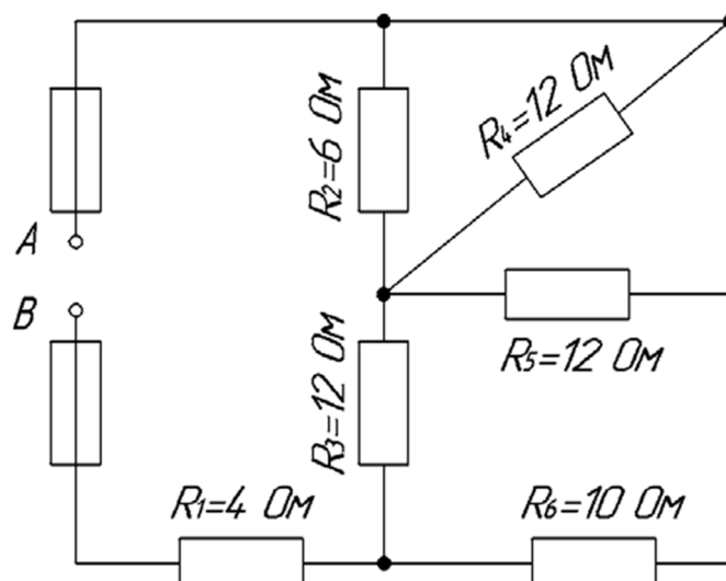
Рисунок 7 – Электрическая схема
