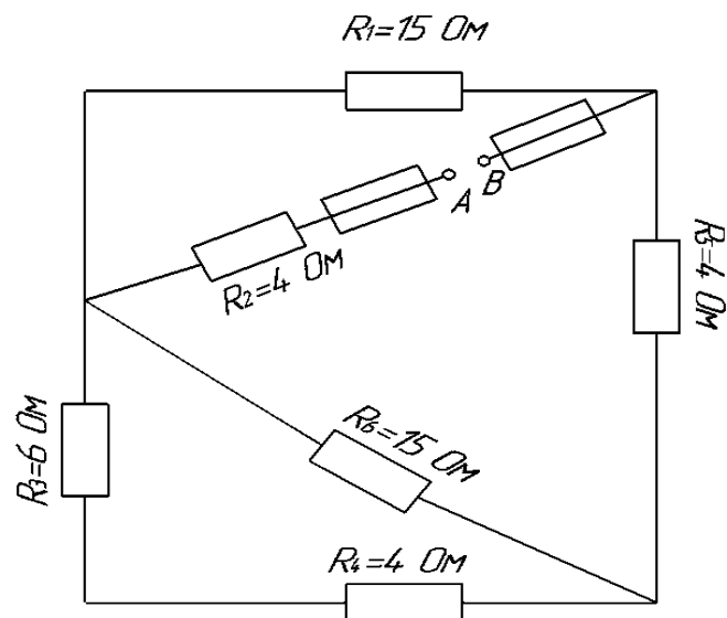
Рисунок 5 – Электрическая схема
