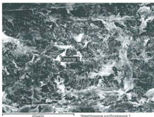
Рисунок 2 – Микроструктура поверхности железо-никель-фосфорного покрытия Figure 2 – Microstructure of the surface of the iron-nickel-phosphorus coating
