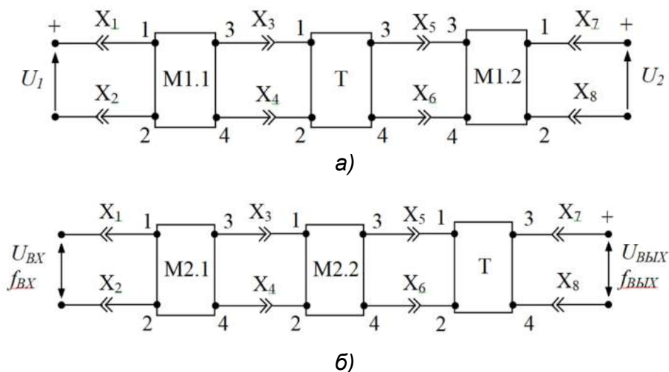
Рисунок 2 – Структурные схемы конвертора (а) и преобразователя частоты (б), выполненные на модульных блоках (рисунок 1)
