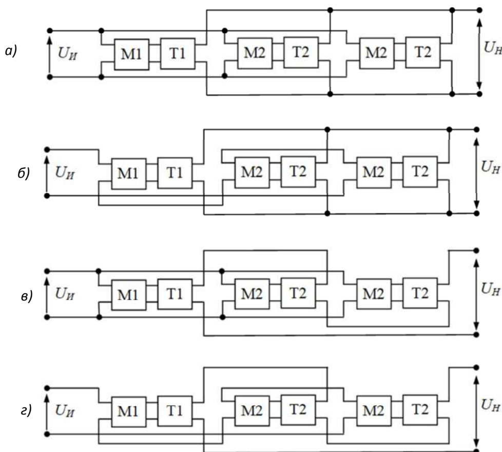
Рисунок 3 – Способы подключения модульных блоков к источнику электроэнергии U_H и нагрузке U_H Figure 3 – Methods for connecting modular units to the power source U_H and load U_H
