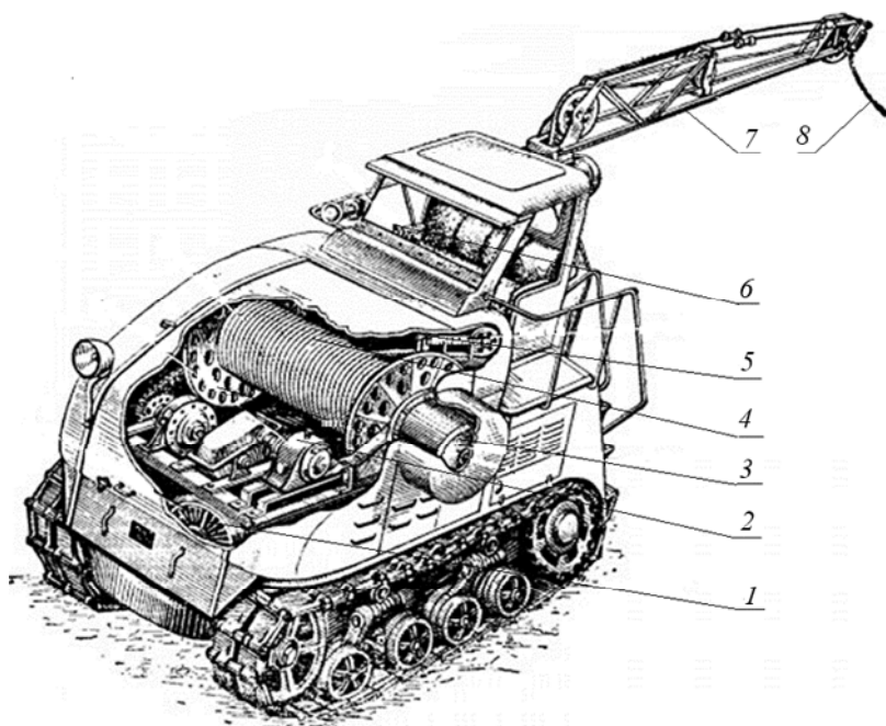
Рисунок 1 – Электротрактор ВИМЭ-2:
