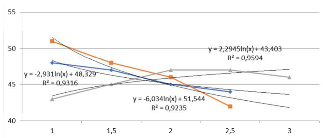
Рисунок 5 – Изменение угла поворота грядиля от скорости движения агрегата
