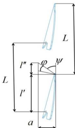
Рисунок 4 – Определение зоны деформации почвы перед рабочим органом в продольном направлении: l' – конструктивный параметр, характеризующий продольный размер (длину) рабочего органа «Скат» (вылет стойки) в проекции на продольно-горизонтальную плоскость, м; l'' – зона деформации почвы в продольном направлении, м; \beta, \varphi, \rho, \psi – углы соответственно крошения, внешнего и внутреннего трения, сдвига (скола) почвы, град
