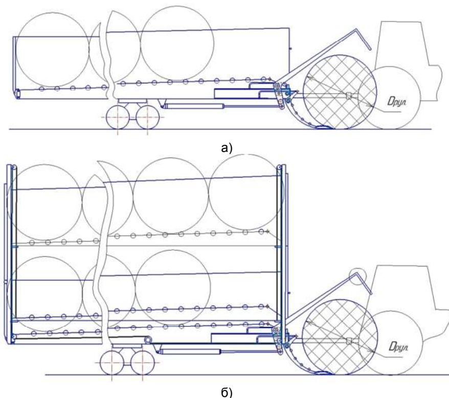
Рисунок 3 – Схемы погрузчиков-транспортировщиков рулонов сена ПТРС-1 (а) и ПТРС-2 (б) / Figure 3 – Schemes of loaders-transporters of hay rolls PRS-1 (a) and PTS-2 (b)
