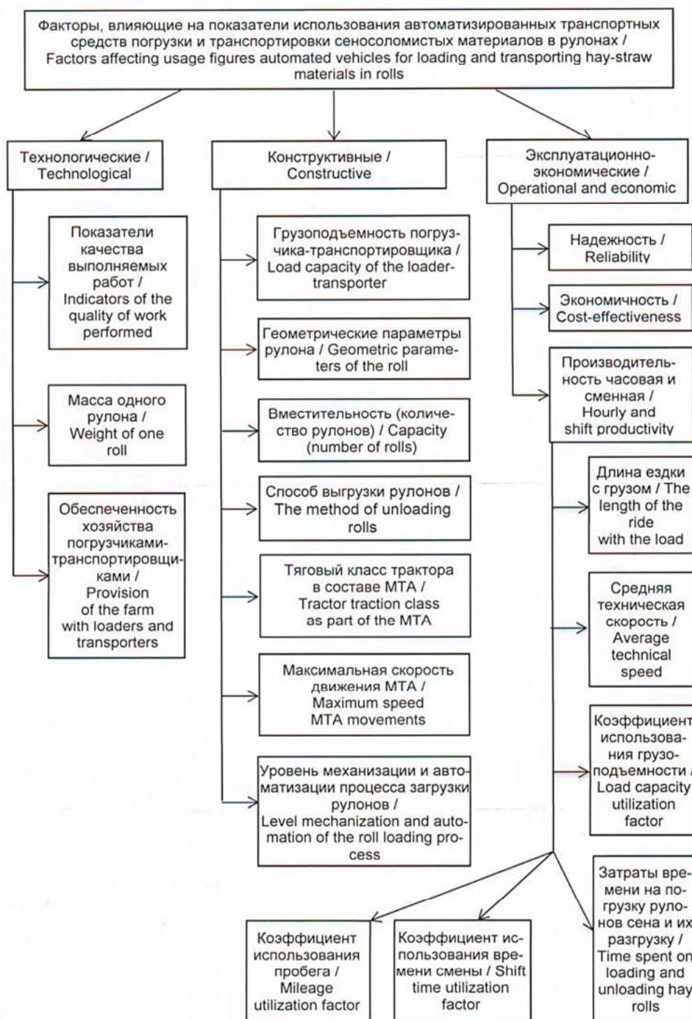
Рисунок 4 – Факторы, влияющие на показатели использования автоматизированных транспортных средств погрузки и транспортировки сеносоломистых материалов в рулонах Figure 4 – Factors affecting usage figures automated vehicles for loading and transporting hay-straw materials in rolls
