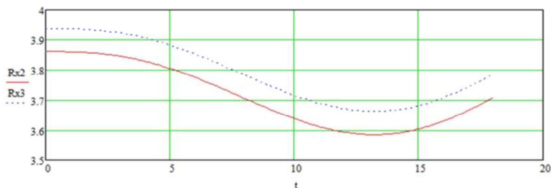
Рисунок 3 – Зависимость касательных реакций R_{x2} , R_{x3} (Н) опорной поверхности на грунте суглинок при перемещении шагающим способом экспериментального транспортного средства
