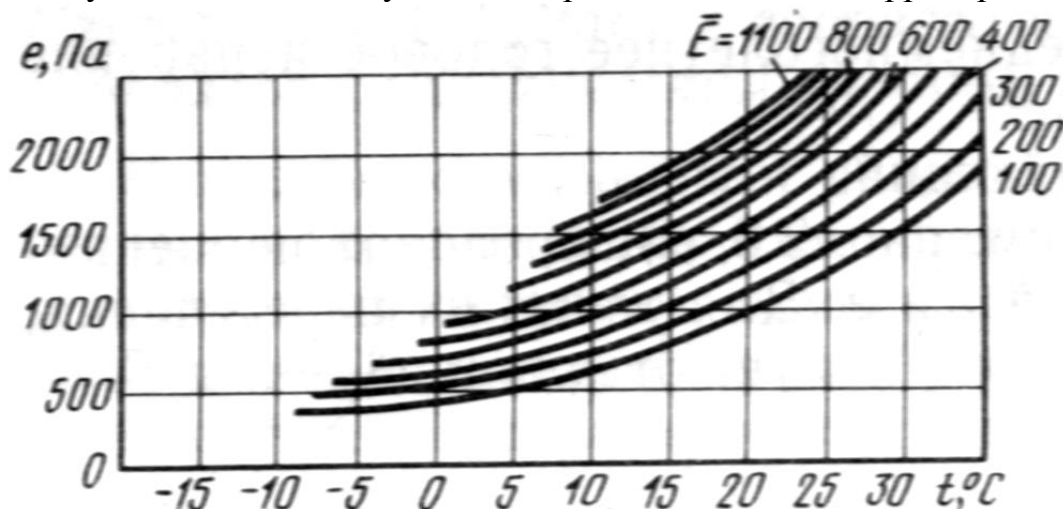
Рис. 1. Номограмма для вычисления среднегодового испарения по методу Р.А. Константинова
