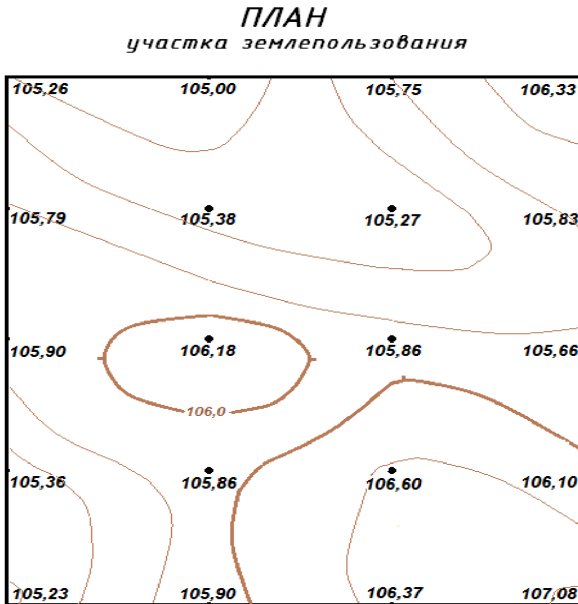
1:1000 высота сечения рельефа 0,25 м Рисунок 10 – Топографический план участка
