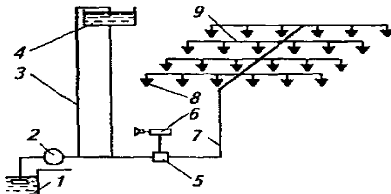
Рисунок 2 - Схема водяной спринклерной установки:
