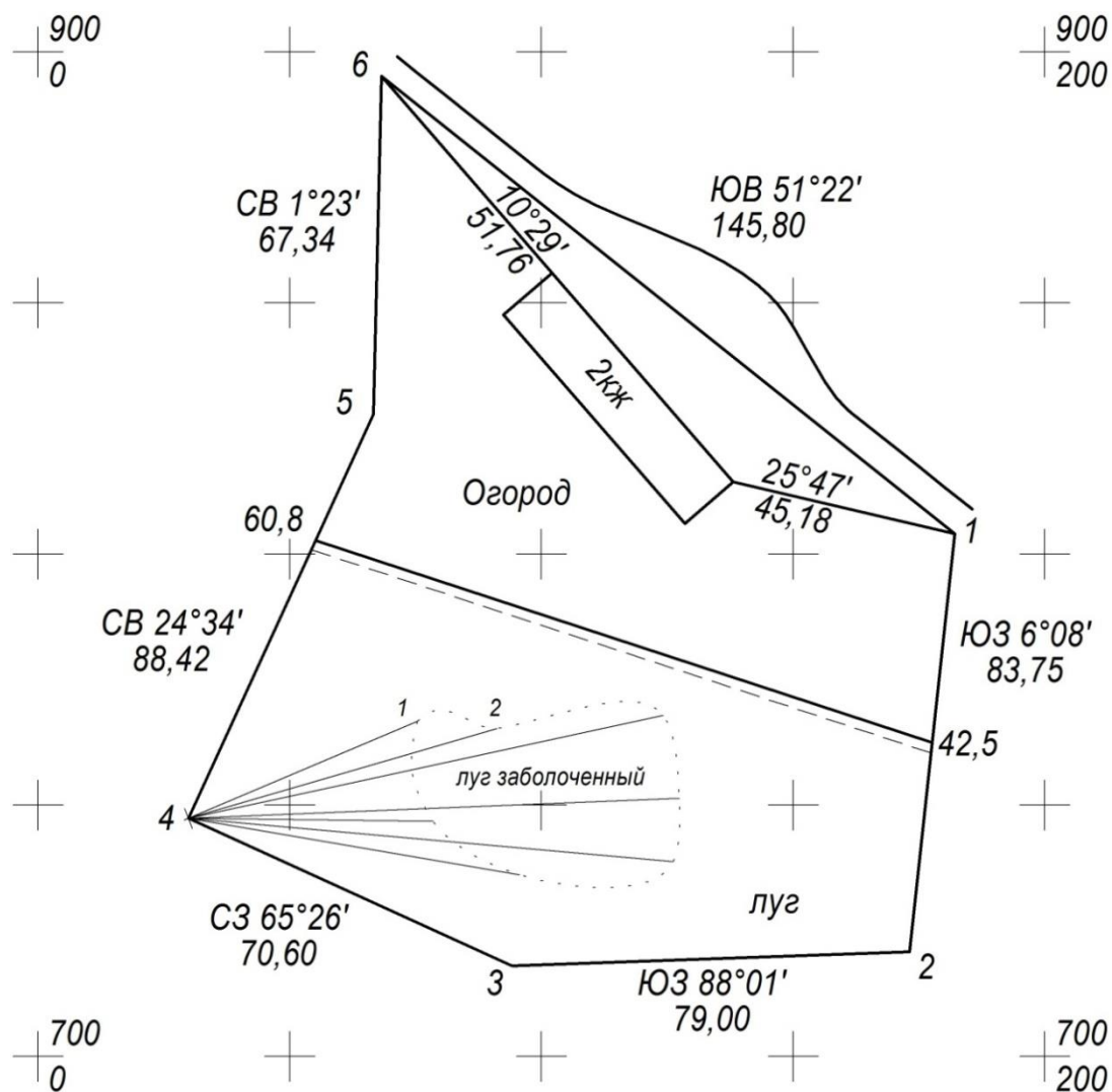
Рисунок 3 – Абрис теодолитной съёмки
