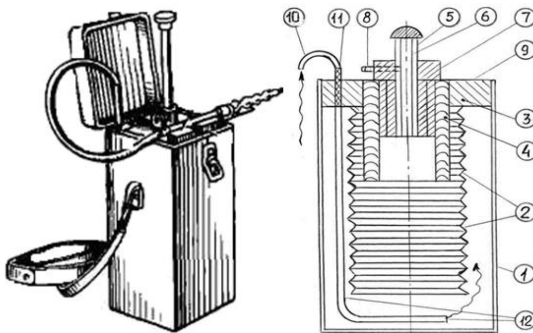
Рисунок 1 - Газоанализатор УГ-2
