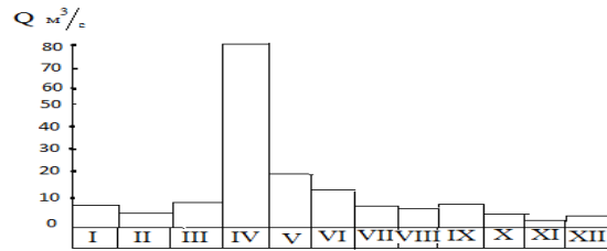
Рис. 3. Расчетный гидрограф
