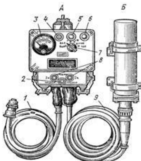
Рисунок 2 – Рентгенометр ДП-3Б
