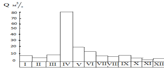
Рис. 3. Расчетный гидрограф
